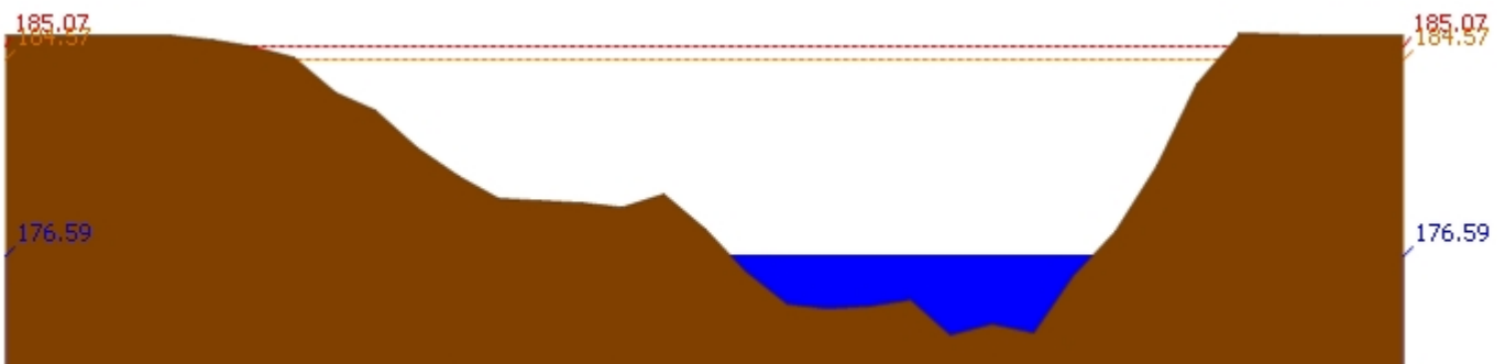
สถานี 070116T แม่น้ำวังที่บ้านแม่เตี๊ยะ ต.แม่ถอด อ.เถิน จ.ลำปาง ระดับน้ำ 176.59 ม.รทก.
