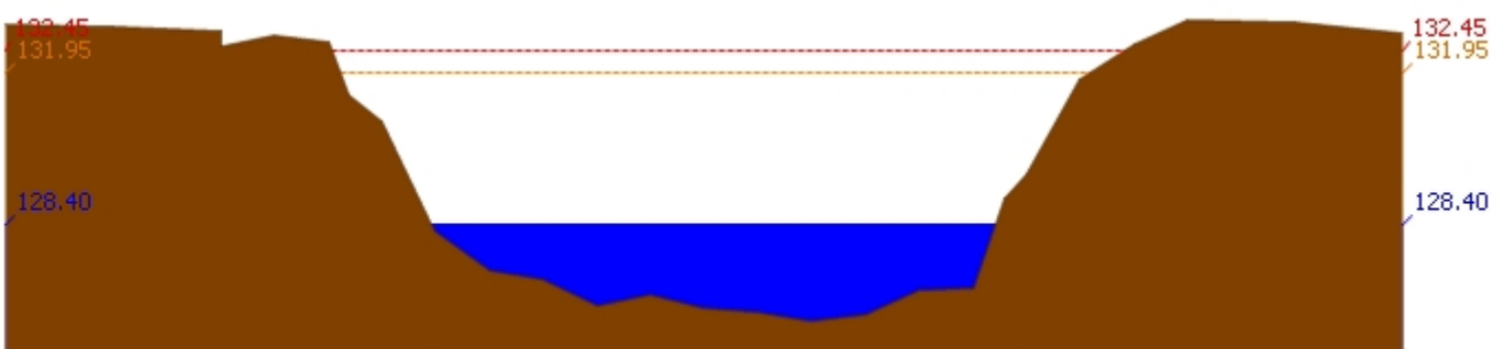
สถานี 070118T แม่น้ำวังที่บ้านแม่สลิด ต.แม่สลิด อ.บ้านตาก จ.ตาก ระดับน้ำ 128.40 ม.รทก.
