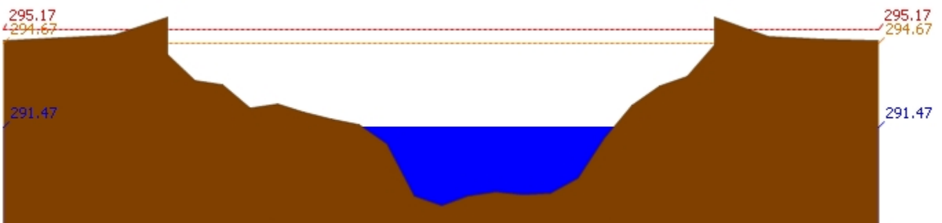
สถานี 060709T น้ำแม่กวงที่ลำพูน ต.เวียงของ อ.เมือง จ.ลำพูน ระดับน้ำ 291.47 ม.รทก.
