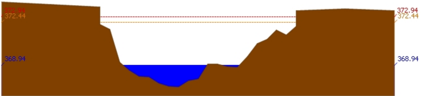
สถานี 060109T แม่น้ำปิงที่บ้านสบอ้อ ต.แม่ระ อ.เชียงดาว จ.เชียงใหม่ ระดับน้ำ 368.94 ม.รทก.
