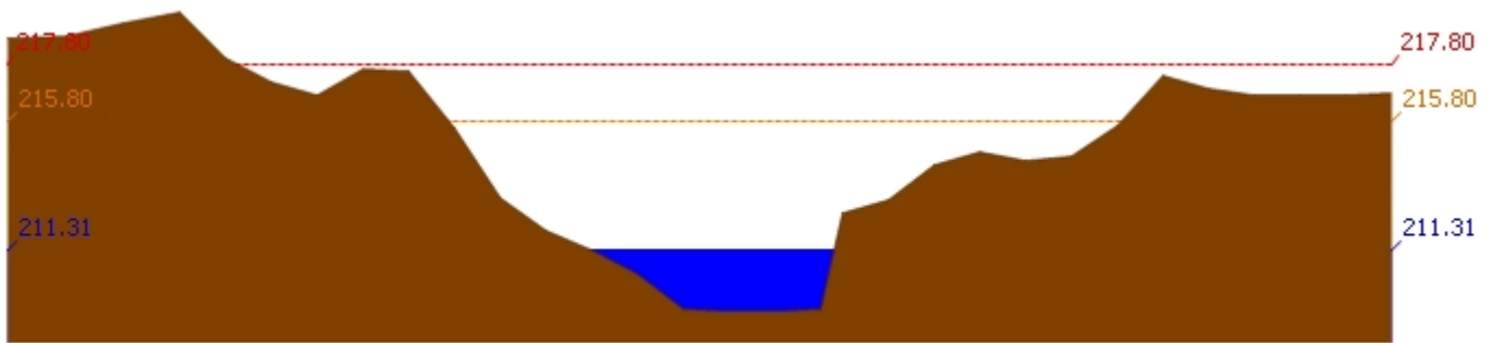
สถานี 120205T แม่น้ำป่าสักที่บ้านอู่กระทัด ต.ศิลา อ.หล่มเก่า จ.เพชรบูรณ์ ระดับน้ำ 211.31 ม.รทก.
