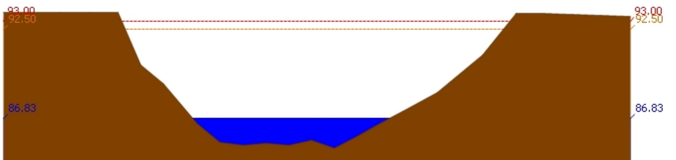
สถานี 120110T แม่น้ำป่าสักที่บ้านวังโบสถ์ ต.วังโบสถ์ อ.หนองไผ่ จ.เพชรบูรณ์ ระดับน้ำ 86.83 ม.รทก.
