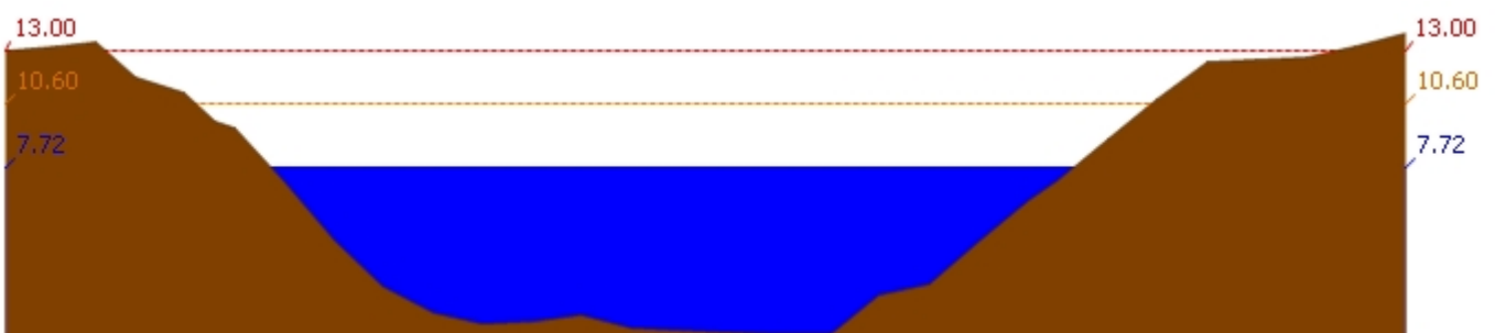
สถานี 120106T แม่น้ำป่าสักที่ อ.เสนาห์ ต.ศาลาวิไทย อ.เสนาห์ จ.สระบุรี ระดับน้ำ 7.72 ม.รทก.
