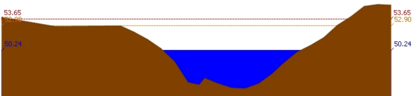
สถานี 120113T แม่น้ำป่าสักที่บ้านเขาค้าง ต.คลองกระจิง อ.ศรีเทพ จ.เพชรบูรณ์ ระดับน้ำ 50.24 ม.รทก.
