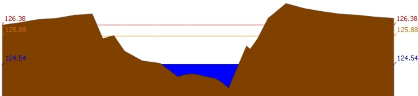
สถานี 110301T คลองโพธิ์ที่บ้านคลองบัวงามสามัคคี ต.ปางสวรรค์ อ.ชุมตาบง จ.นครสวรรค์ ระดับน้ำ 124.54 ม.รทก.
