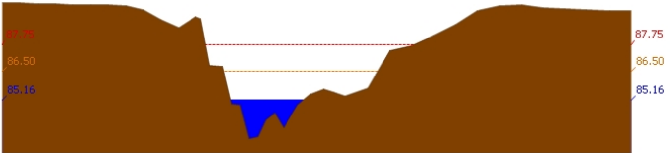
สถานี 110403T หัวขั้วเขลาที่บ้านดินแดง ต.ประตู่ยืน อ.ลานสัก จ.อุทัยธานี ระดับน้ำ 85.16 ม.รทก.
