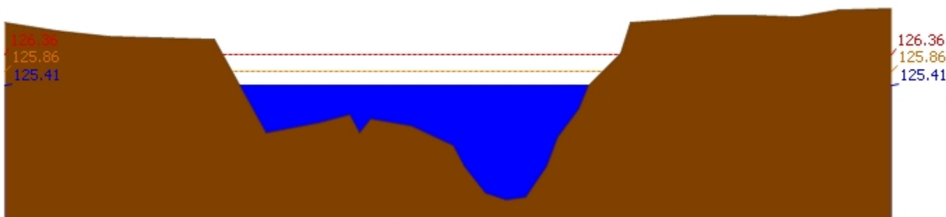
สถานี 110401T หัวขั้วทึบเสลาที่บ้านบึงอ้ายเจียม ต.ระบำ อ.ลานสัก จ.อุทัยธานี ระดับน้ำ 125.41 ม.รทก.
