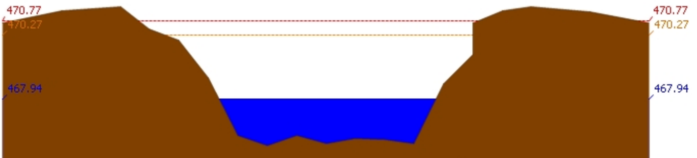
สถานี 061206T น้ำแม่แจ่มที่บ้านทัพ ต.ท่าผา อ.แม่แจ่ม จ.เชียงใหม่ ระดับน้ำ 467.94 ม.รทก.
