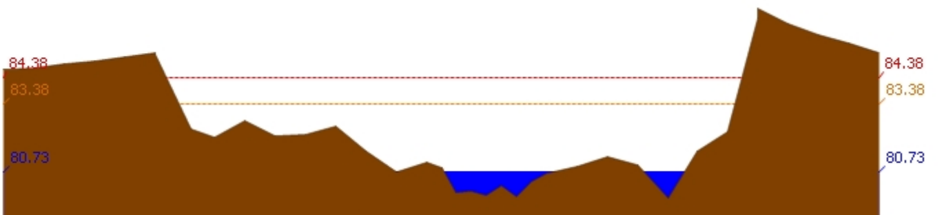
สถานี 062001T คลองสวนหมากที่บ้านน้ำไทรง ต.ท่าขุนราม อ.เมือง จ.กำแพงเพชร ระดับน้ำ 80.73 ม.รทก.
