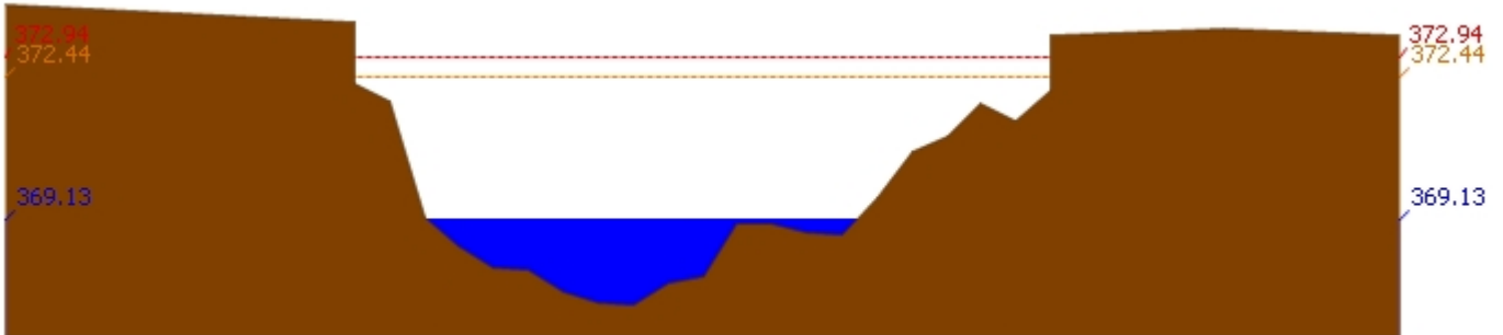
สถานี 060109T แม่น้ำปิงที่บ้านสบอ้อ ต.แม่ระ อ.เชียงดาว จ.เชียงใหม่ ระดับน้ำ 369.13 ม.รทก.
