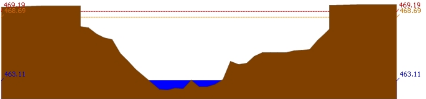
สถานี 060905T น้ำแม่ลี้ที่อำเภอเถิน ต.ลี้ อ.ลี้ จ.ลำพูน ระดับน้ำ 463.11 ม.รทก.
