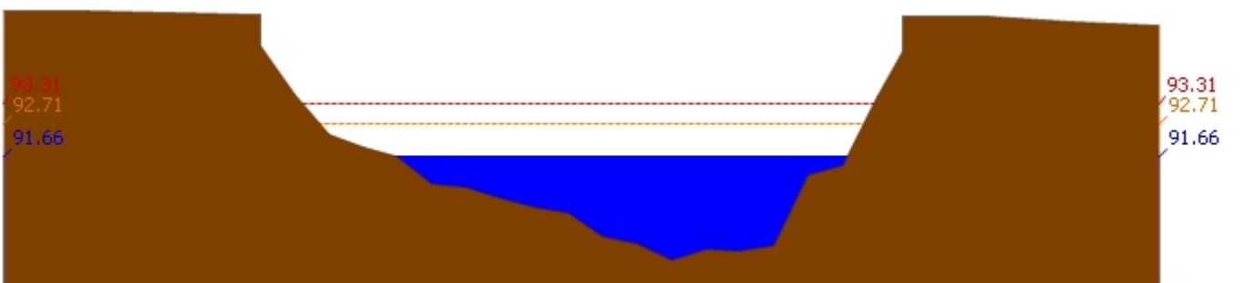
สถานี 061901T คลองแม่ระกาที่บ้านวังชะโอน ต.ท่าไม้ อ.พรานกระต่าย จ.กำแพงเพชร ระดับน้ำ 91.66 ม.รทก.
