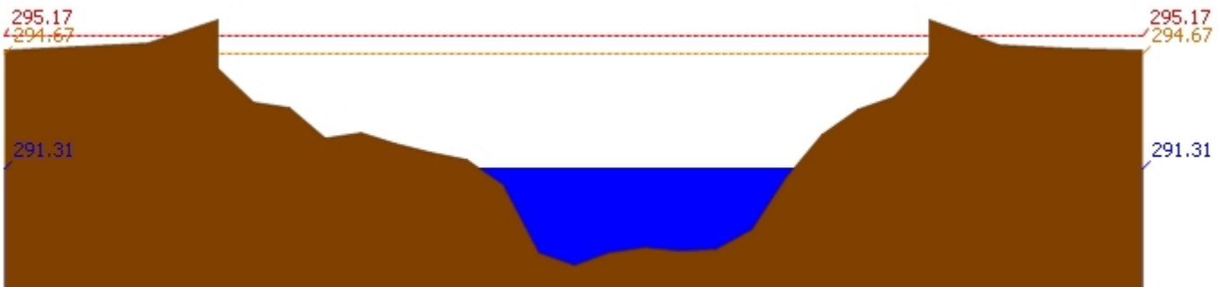
สถานี 060709T น้ำแม่กวังที่ลำพูน ต.เวียงของ อ.เมือง จ.ลำพูน ระดับน้ำ 291.31 ม.รทก.
