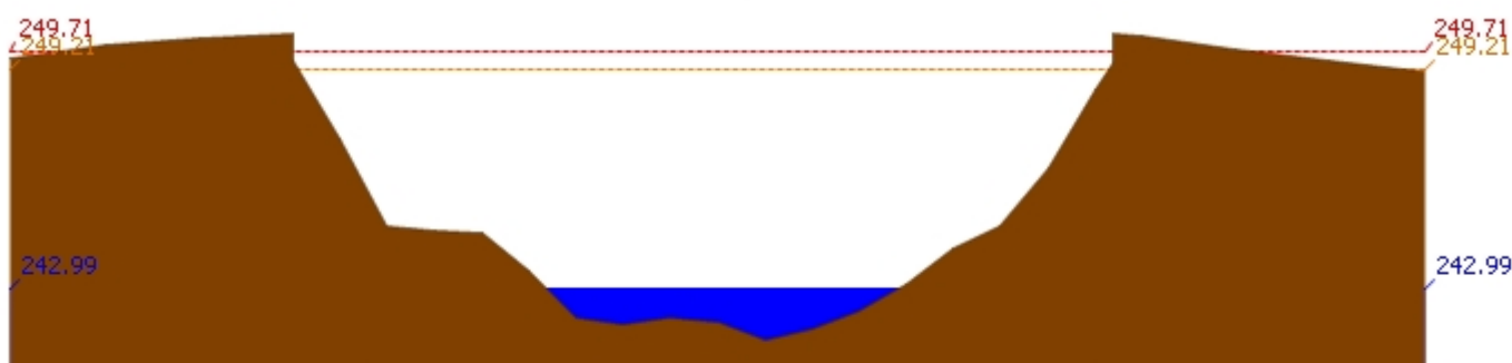
สถานี 070112T แม่น้ำวังที่บ้านบุญนาค ต.บุญนาคพัฒนา อ.เมืองลำปาง จ.ลำปาง ระดับน้ำ 242.99 ม.รทก.
