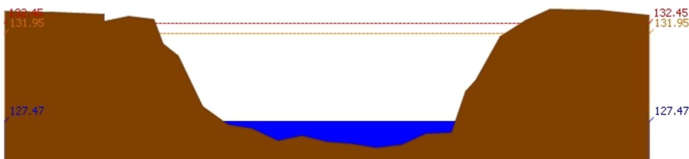
สถานี 070118T แม่น้ำวังที่บ้านแม่สลิด ต.แม่สลิด อ.บ้านตาก จ.ตาก ระดับน้ำ 127.47 ม.รทก.
