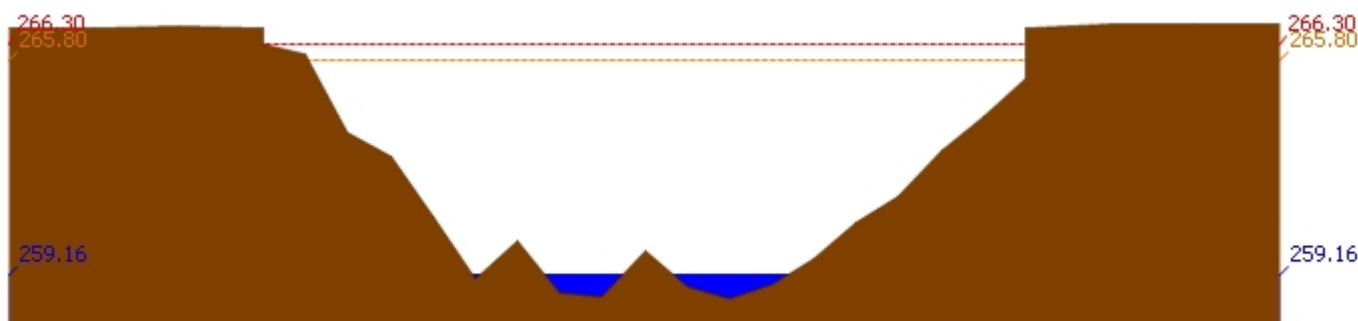
สถานี 070604T น้ำแม่จางที่บ้านสุโหมโขมมงคล ต.หัวเสือ อ.แม่ทะ จ.ลำปาง ระดับน้ำ 259.16 ม.รทก.
