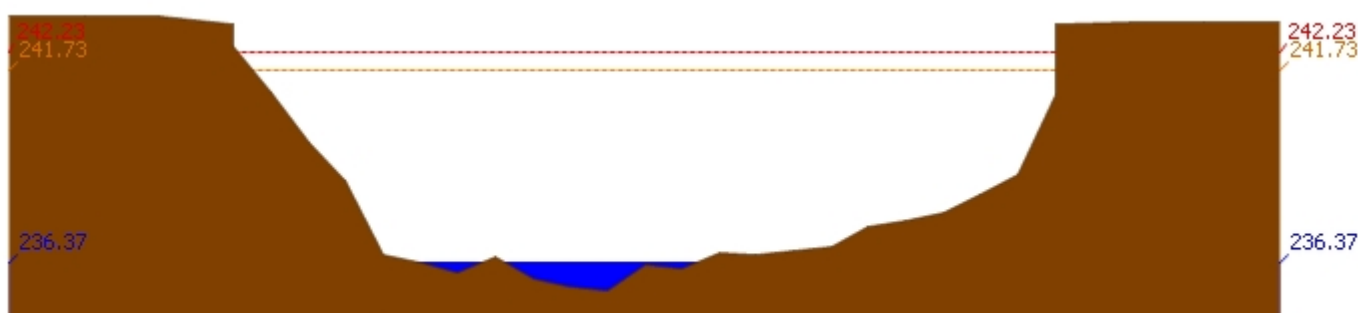
สถานี 070114T แม่น้ำวังที่บ้านปางชัย ต.บ้านเสด็จ อ.เมืองลำปาง จ.ลำปาง ระดับน้ำ 236.37 ม.รทก.
