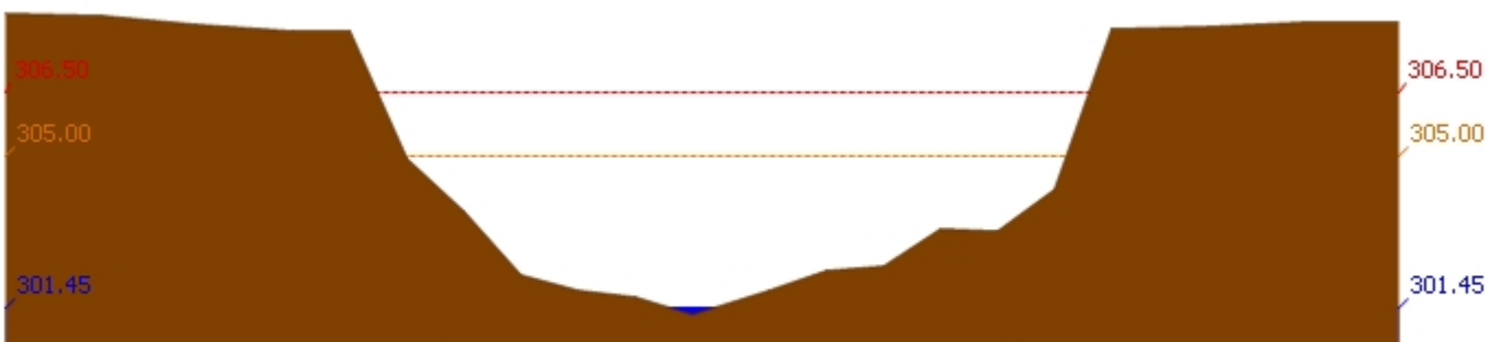
สถานี 120304T ห้วยน้ำพุที่บ้านกกกะบาก ต.โป่ง อ.ด่านซ้าย จ.เลย ระดับน้ำ 301.45 ม.รทก.
