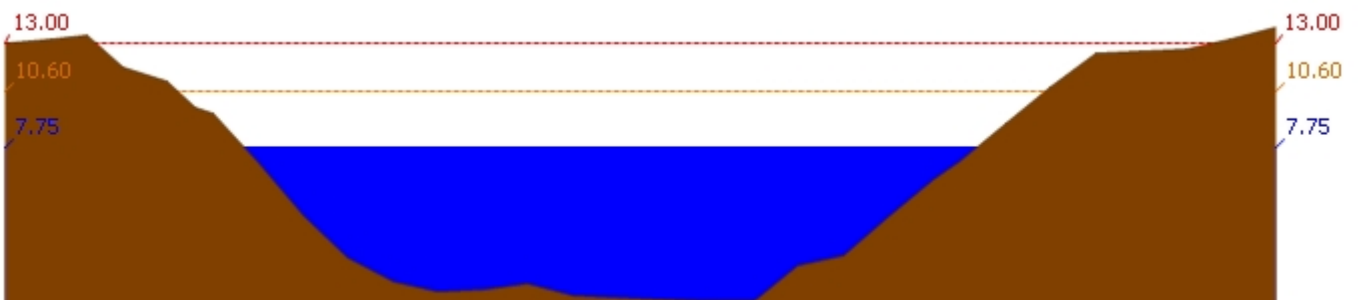
สถานี 120106T แม่น้ำป่าสักที่ อ.เสนาห์ ต.ศาลาวิไทย อ.เสนาห์ จ.สระบุรี ระดับน้ำ 7.75 ม.รทก.
