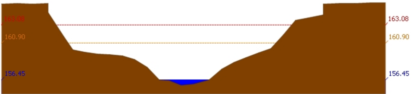
สถานี 120105T แม่น้ำป่าสักที่บ้านวังมเสหนือ ต.ทำอิบุญ อ.หล่มสัก จ.เพชรบูรณ์ ระดับน้ำ 156.45 ม.รทก.
