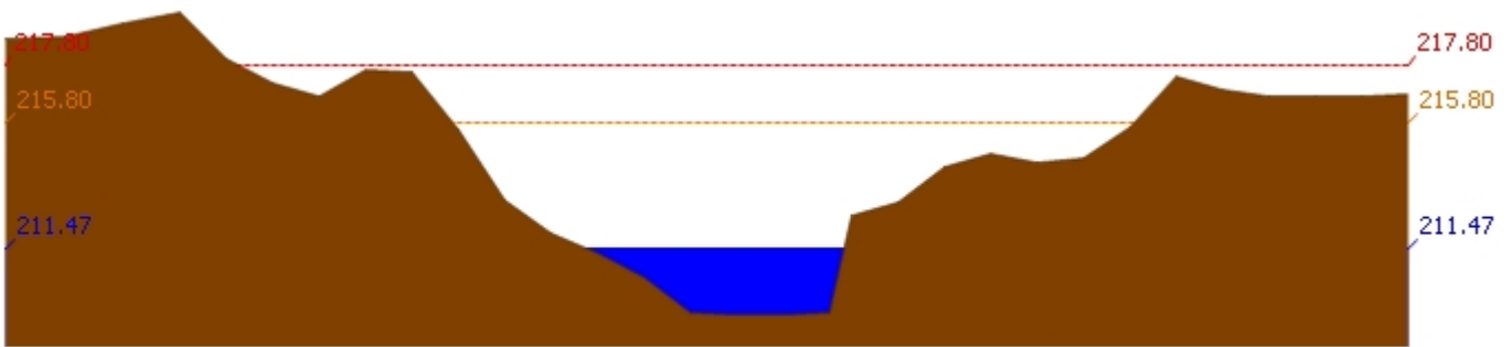
สถานี 120205T แม่น้ำป่าสักที่บ้านอู่กะทาด ต.ศิลา อ.หล่มเก่า จ.เพชรบูรณ์ ระดับน้ำ 211.47 ม.รทก.
