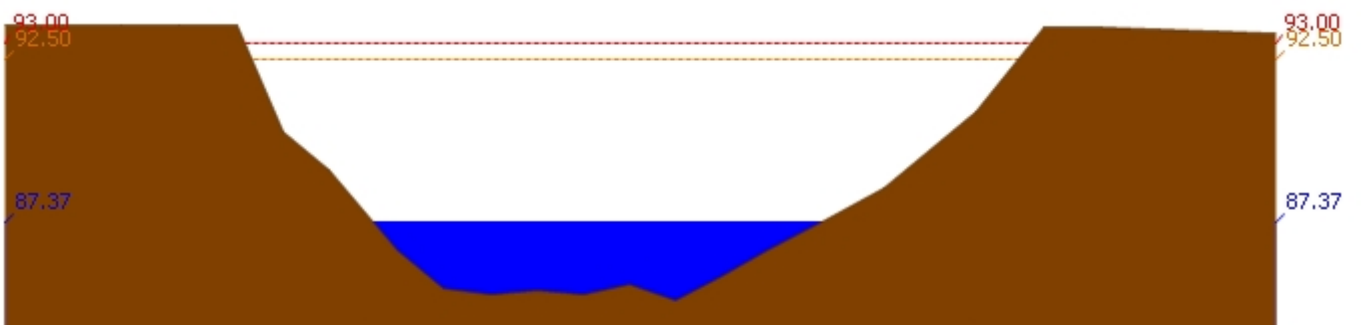
สถานี 120110T แม่น้ำป่าสักที่บ้านวังโบสถ์ ต.วังโบสถ์ อ.หนองไผ่ จ.เพชรบูรณ์ ระดับน้ำ 87.37 ม.รทก.
