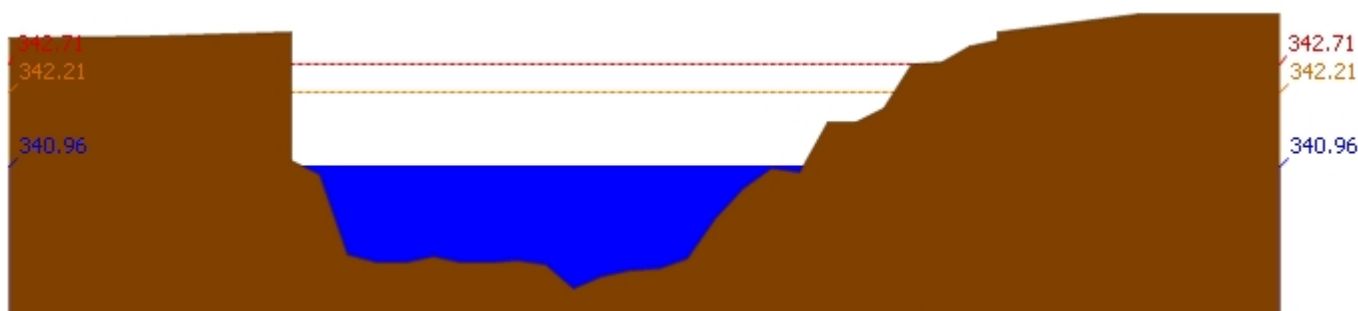
สถานี 070304T น้ำแม่สอยที่บ้านหนองกอก ต.แม่สวก อ.แจ้ห่ม จ.ลำปาง ระดับน้ำ 340.96 ม.รทก.
