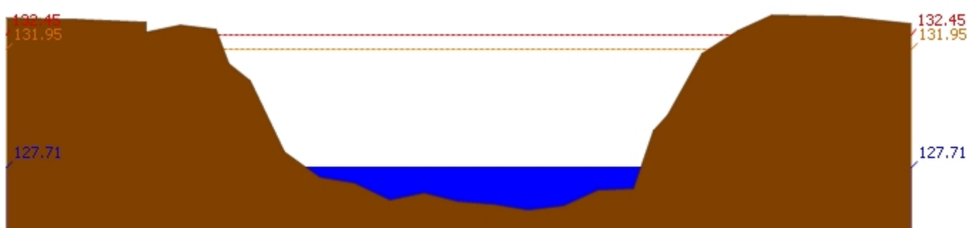
สถานี 070118T แม่น้ำวังที่บ้านแม่สลิด ต.แม่สลิด อ.บ้านตาก จ.ตาก ระดับน้ำ 127.71 ม.รทก.
