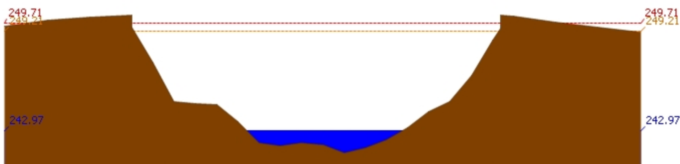
สถานี 070112T แม่น้ำวังที่บ้านบุญนาคร ต.บุญนาครพัฒนา อ.เมืองลำปาง จ.ลำปาง ระดับน้ำ 242.97 ม.รทก.
