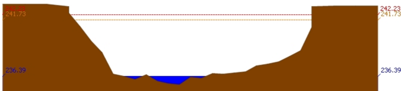
สถานี 070114T แม่น้ำวังที่บ้านปางชัย ต.บ้านเสด็จ อ.เมืองลำปาง จ.ลำปาง ระดับน้ำ 236.39 ม.รทก.
