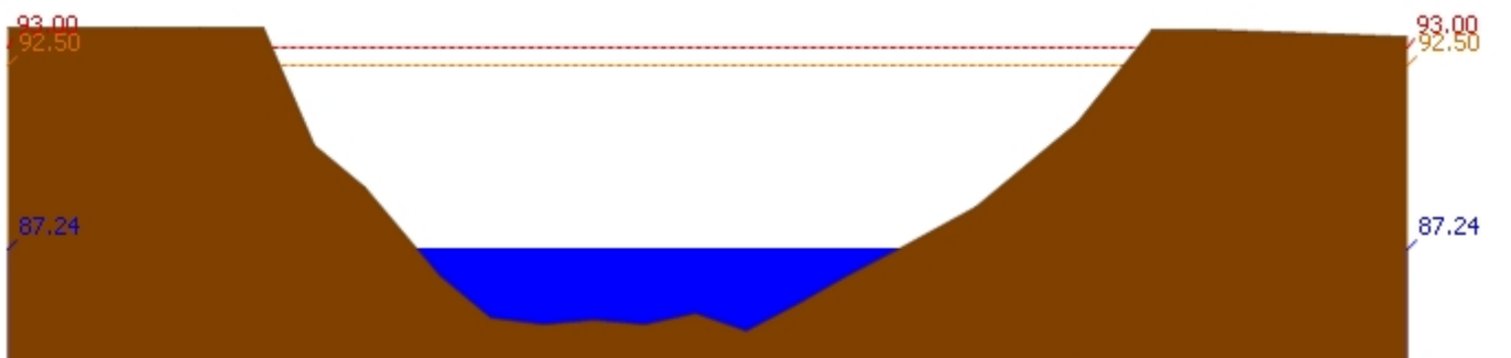
สถานี 120110T แม่น้ำป่าสักที่บ้านวังโบสถ์ ต.วังโบสถ์ อ.หนองไผ่ จ.เพชรบูรณ์ ระดับน้ำ 87.24 ม.รทก.
