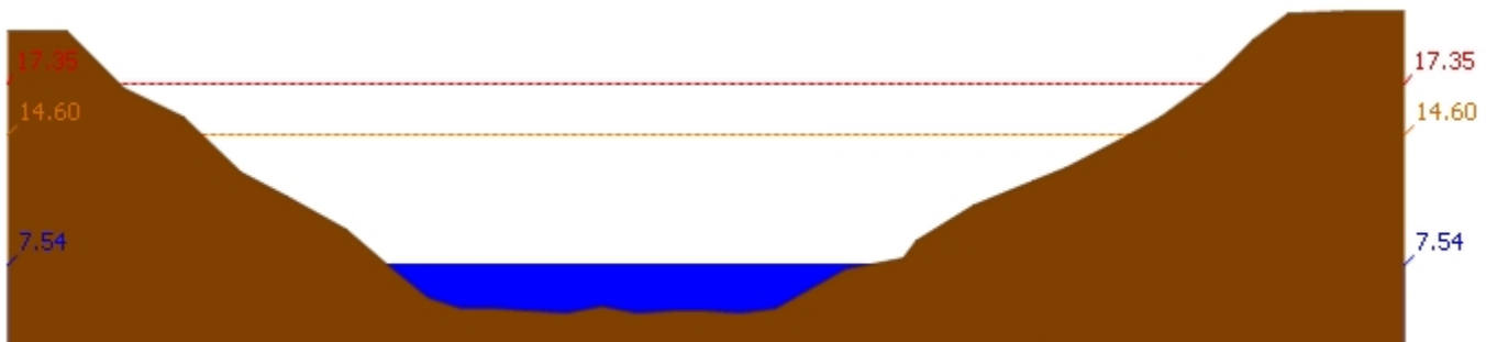
สถานี 120109T แม่น้ำป่าสักที่ อ.แก่งค้อย ต.แก่งค้อย อ.แก่งค้อย จ.สระบุรี ระดับน้ำ 7.54 ม.รทก.
