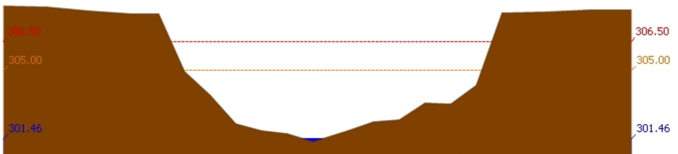
สถานี 120304T ห้วยน้ำพุงที่บ้านกกกะบาก ต.โป่ง อ.ด่านซ้าย จ.เลย ระดับน้ำ 301.46 ม.รทก.
