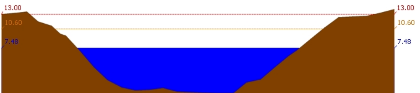
สถานี 120106T แม่น้ำป่าสักที่ อ.เสนาห์ ต.ศาลาวิไทย อ.เสนาห์ จ.สระบุรี ระดับน้ำ 7.48 ม.รทก.
