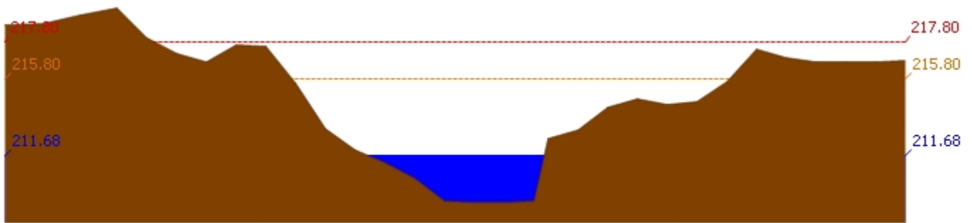
สถานี 120205T แม่น้ำป่าสักที่บ้านอู่กะทาด ต.ศิลา อ.หล่มเก่า จ.เพชรบูรณ์ ระดับน้ำ 211.68 ม.รทก.
