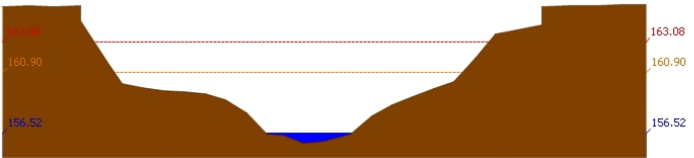
สถานี 120105T แม่น้ำป่าสักที่บ้านวังมเหนื่อ ต.ทำอัญญา อ.หล่มสัก จ.เพชรบูรณ์ ระดับน้ำ 156.52 ม.รทก.
