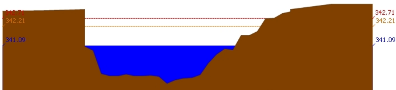
สถานี 070304T น้ำแม่สอยที่บ้านหนองกอก ต.แม่สกก อ.แจ้ห่ม จ.ลำปาง ระดับน้ำ 341.09 ม.รทก.
