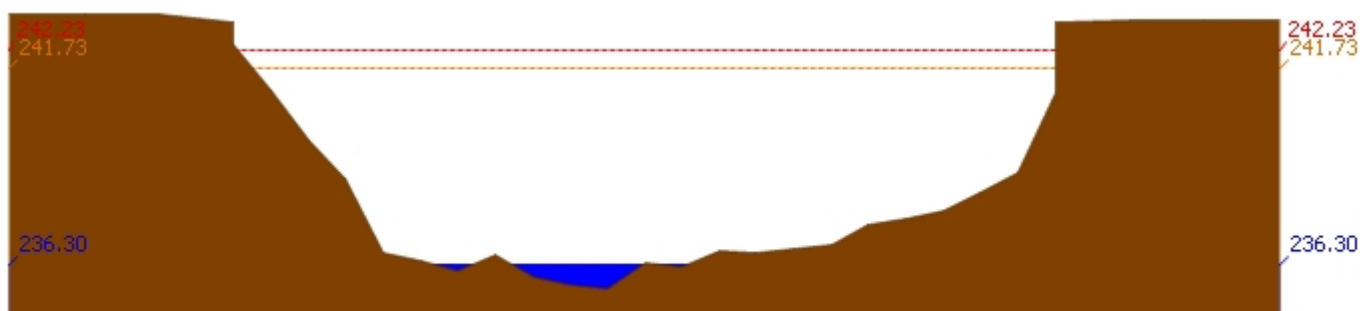
สถานี 070114T แม่น้ำวังที่บ้านปางชัย ต.บ้านเสด็จ อ.เมืองลำปาง จ.ลำปาง ระดับน้ำ 236.30 ม.รทก.
