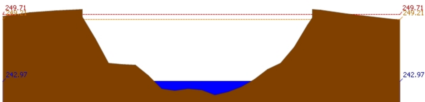
สถานี 070112T แม่น้ำวังที่บ้านบุญนาค ต.บุญนาคพัฒนา อ.เมืองลำปาง จ.ลำปาง ระดับน้ำ 242.97 ม.รทก.
