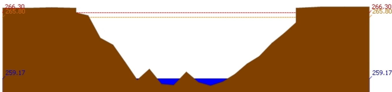
สถานี 070604T น้ำแม่จางที่บ้านสุโหมโขมมงคล ต.หัวเสือ อ.แม่ทะ จ.ลำปาง ระดับน้ำ 259.17 ม.รทก.
