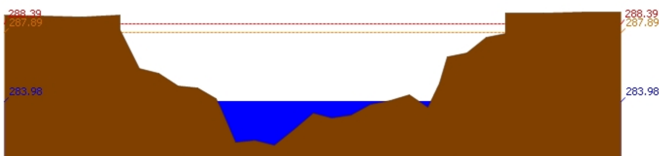
สถานี 070111T แม่บัววังที่บ้านแปงโปงชัย ต.บ้านเสา อ.แจ้ห่ม จ.ลำปาง ระดับน้ำ 283.98 ม.รทก.
