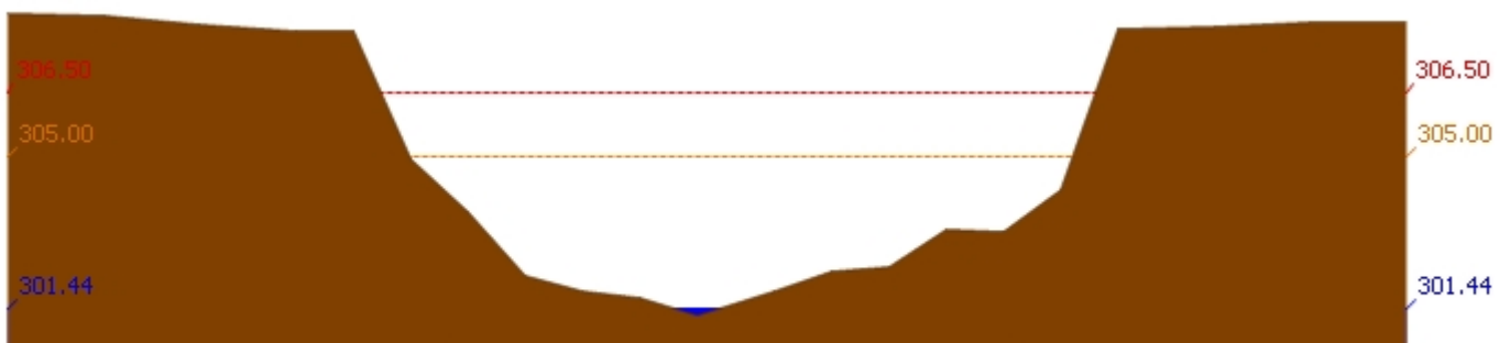
สถานี 120304T ห้วยน้ำพุที่บ้านกกกะบาก ต.โป่ง อ.ด่านซ้าย จ.เลย ระดับน้ำ 301.44 ม.รทก.
