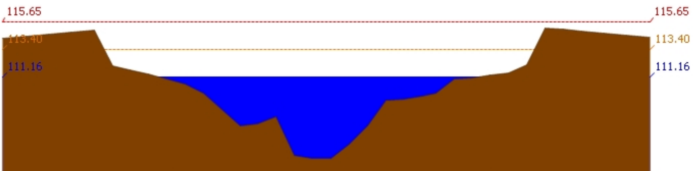
สถานี 120107T แม่น้ำป่าสักที่ อ.เมืองเพชรบูรณ์ ต.นาป่า อ.เมือง จ.เพชรบูรณ์ ระดับน้ำ 111.16 ม.รทก.
