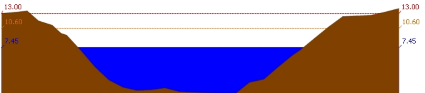
สถานี 120106T แม่น้ำป่าสักที่ อ.เสนาไห้ ต.ศาลาวิไทย อ.เสนาไห้ จ.สระบุรี ระดับน้ำ 7.45 ม.รทก.
