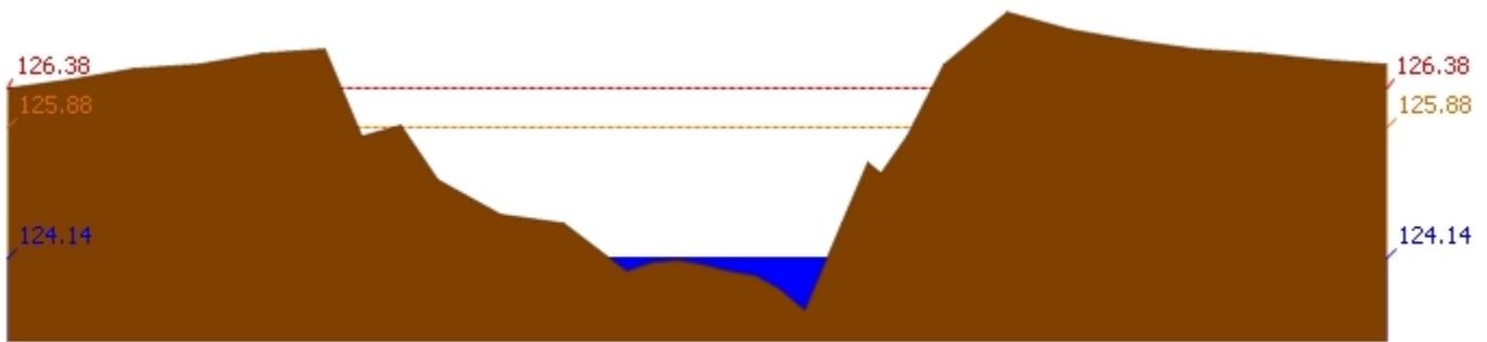
สถานี 110301T คลองโพธิ์ที่บ้านคลองบัวสามัคคี ต.ปางสวรรค์ อ.ชุมตาบง จ.นครสวรรค์ ระดับน้ำ 124.14 ม.รทก.
