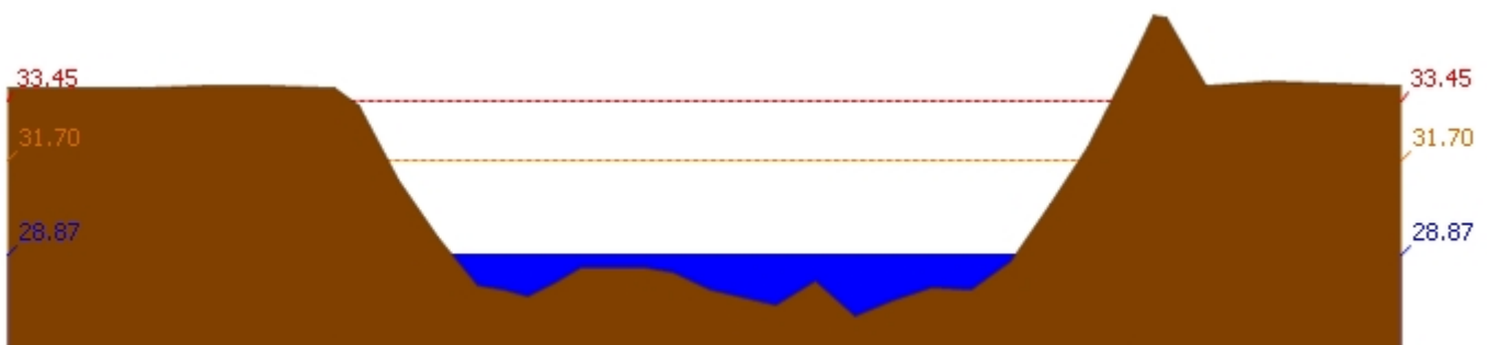
สถานี 110503T แม่น้ำตากแดดที่บ้านหนองขาลาย ต.หนองหลวง อ.สว่างอารมณ์ จ.อุทัยธานี ระดับน้ำ 28.87 ม.รทก.
