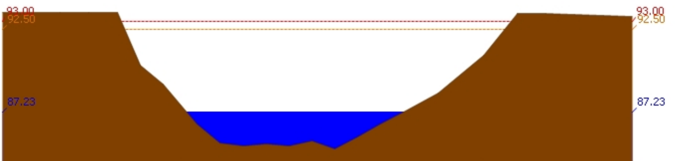
สถานี 120110T แม่น้ำป่าสักที่บ้านวังโบสถ์ ต.วังโบสถ์ อ.หนองไผ่ จ.เพชรบูรณ์ ระดับน้ำ 87.23 ม.รทก.
