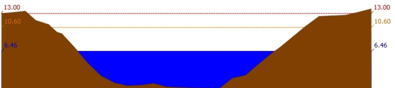
สถานี 120106T แม่น้ำป่าสักที่ อ.เสาไห้ ต.ศาลาวิไทย อ.เสาไห้ จ.สระบุรี ระดับน้ำ 6.46 ม.รทก.
