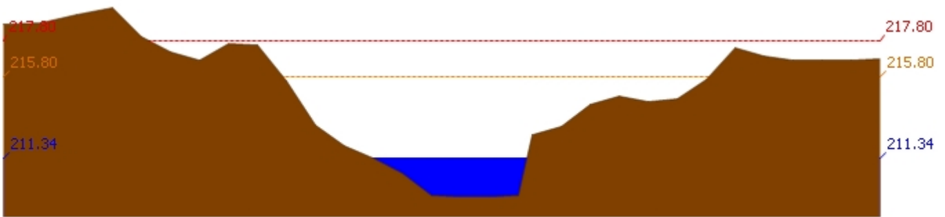
สถานี 120205T แม่น้ำป่าสักที่บ้านอู่กระทัด ต.ศิลา อ.หล่มเก่า จ.เพชรบูรณ์ ระดับน้ำ 211.34 ม.รทก.
