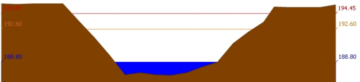
สถานี 120901T ห้วยมวกเหล็กที่ อ.มวกเหล็ก ต.มวกเหล็ก อ.มวกเหล็ก จ.สระบุรี ระดับน้ำ 188.80 ม.รทก.
