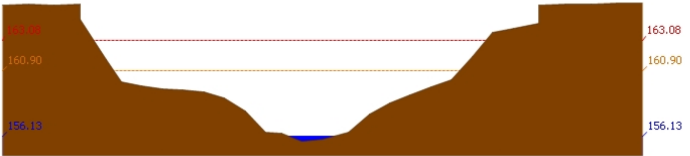
สถานี 120105T แม่น้ำป่าสักที่บ้านวังมเสเหนือ ต.ทำอิบุญ อ.หล่มสัก จ.เพชรบูรณ์ ระดับน้ำ 156.13 ม.รทก.
