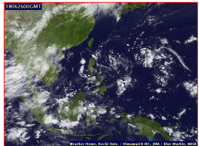
ภาพถ่ายจากดาวเทียม วันที่ ๒๖ มิ.ย. ๒๕๖๑ เวลา ๐๗.๐๐ น.
