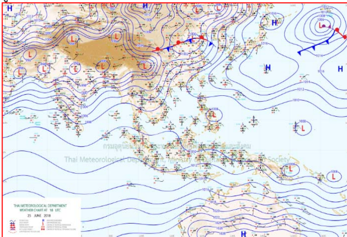
แผนที่อากาศ วันที่ ๒๖ มิ.ย. ๒๕๖๑ เวลา ๐๑.๐๐ น.
