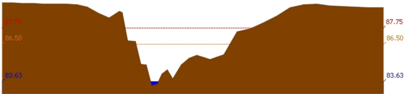
สถานี 110403T ฝายทับเสลาที่บ้านดินแดง ต.ประดู่ป็น อ.ลานสัก จ.อุทัยธานี ระดับน้ำ 83.63 ม.รทก.
