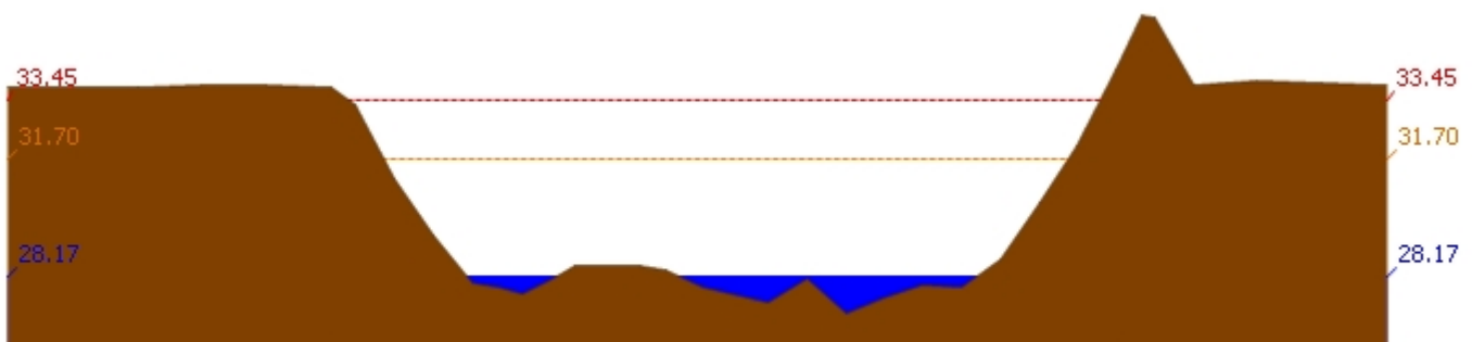
สถานี 110503T ฝ่าน้ำตากแดดที่บ้านหนองชาลาย ต.หนองหลวง อ.สว่างอารมณ์ จ.อุทัยธานี ระดับน้ำ 28.17 ม.รทก.
