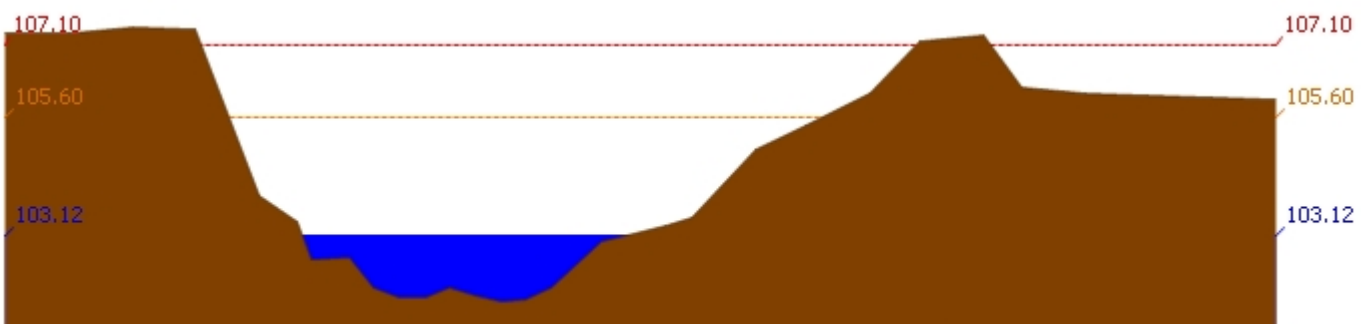
สถานี 110402T ห้วยทับเสลาที่บ้านนาไร่เดียว ต.ลานสัก อ.ลานสัก จ.อุทัยธานี ระดับน้ำ 103.12 ม.รทก.
