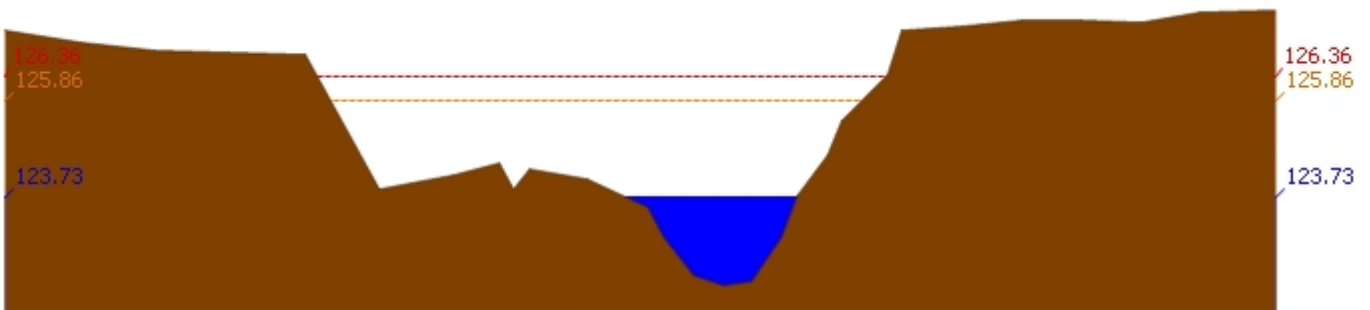
สถานี 110401T ห้วยทับเสลาที่บ้านบึงอ้ายเจียม ต.ระบำ อ.ลานสัก จ.อุทัยธานี ระดับน้ำ 123.73 ม.รทก.
