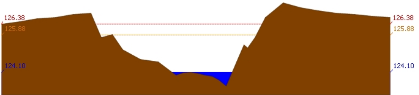
สถานี 110301T คลองโพธิ์ที่บ้านคลองบัวสามัคคี ต.ปางสวรรค์ อ.ชุมตาบง จ.นครสวรรค์ ระดับน้ำ 124.10 ม.รทก.
