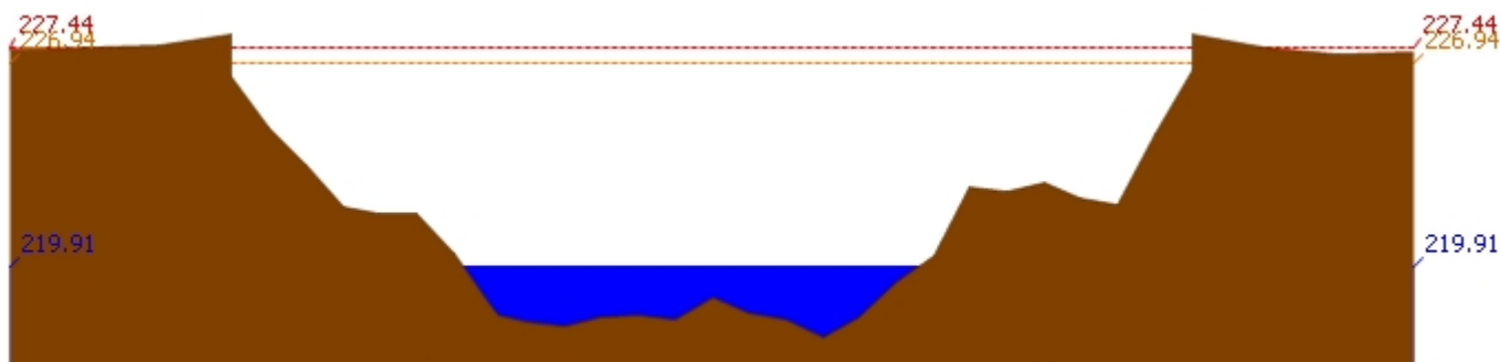
สถานี 070113T แม่น้ำวังที่ จ.ลำปาง ต.เวียงเหนือ อ.เมืองลำปาง จ.ลำปาง ระดับน้ำ 219.91 ม.รทก.
