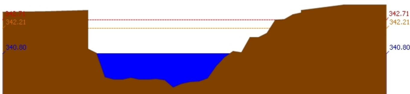
สถานี 070304T น้ำแม่สอยที่บ้านหนองกอก ต.แม่สวก อ.แจ้ห่ม จ.ลำปาง ระดับน้ำ 340.80 ม.รทก.
