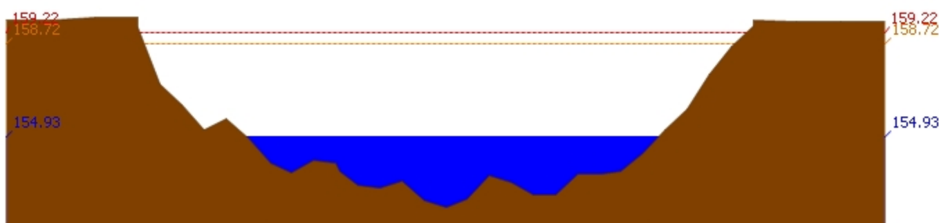
สถานี 070117T แม่น้ำวังที่เทศบาลตำบลแม่ปู ต.แม่ปู อ.แม่พริก จ.ลำปาง ระดับน้ำ 154.93 ม.รทก.
