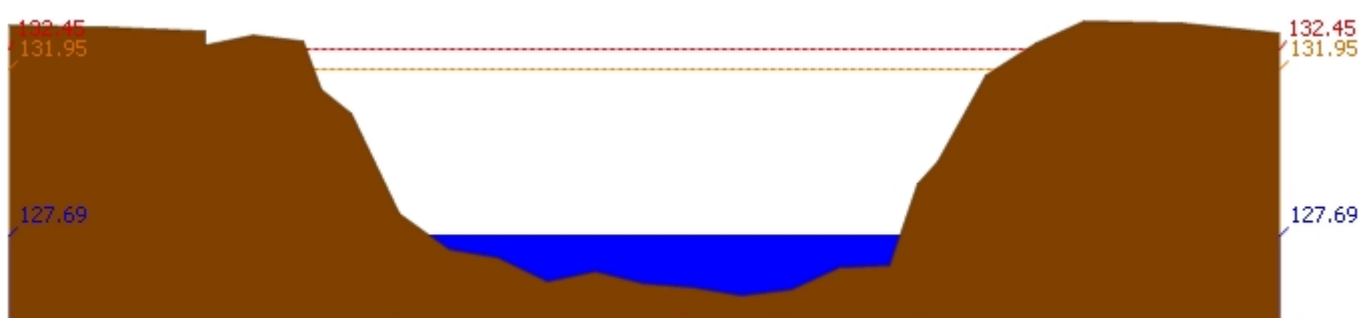
สถานี 070118T แม่น้ำวังที่บ้านแม่สลิด ต.แม่สลิด อ.บ้านตาก จ.ตาก ระดับน้ำ 127.69 ม.รทก.
