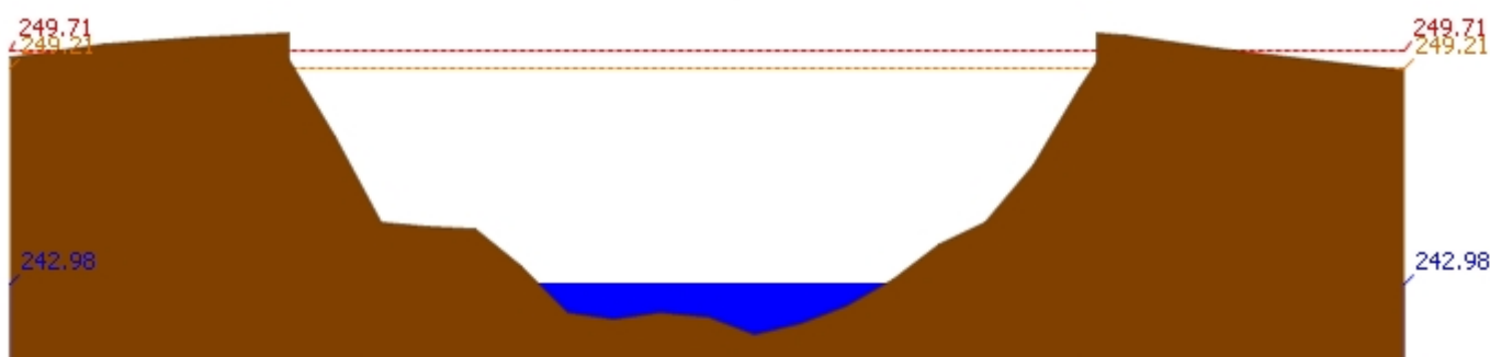
สถานี 070112T แม่น้ำวังที่บ้านบุญนาคร ต.บุญนาครพัฒนา อ.เมืองลำปาง จ.ลำปาง ระดับน้ำ 242.98 ม.รทก.
