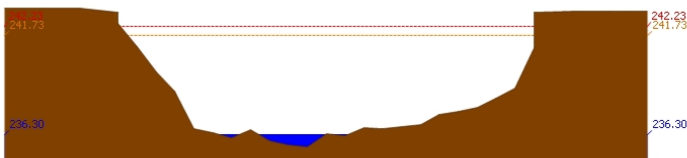
สถานี 070114T แม่น้ำวังที่บ้านปงชัย ต.บ้านเสด็จ อ.เมืองลำปาง จ.ลำปาง ระดับน้ำ 236.30 ม.รทก.
