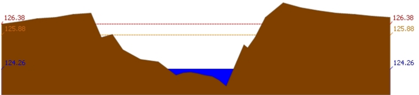
สถานี 110301T คลองโพธิ์ที่บ้านคลองบัวสามัคคี ต.ปางสวรรค์ อ.ชุมตาบง จ.นครสวรรค์ ระดับน้ำ 124.26 ม.รทก.
