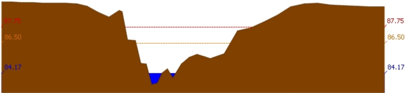
สถานี 110403T หัวขั้วตลับที่บ้านดินแดง ต.ประตู่ยืน อ.ลานสัก จ.อุทัยธานี ระดับน้ำ 84.17 ม.รทก.
