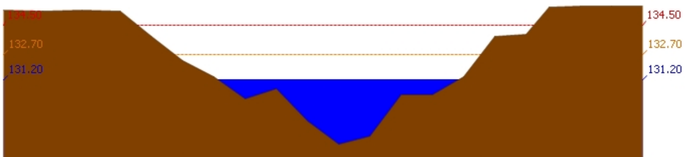
สถานี 120111T แม่น้ำป่าสักที่บ้านจางวาง ต.ลานบ่า อ.หล่มสัก จ.เพชรบูรณ์ ระดับน้ำ 131.20 ม.รทก.
