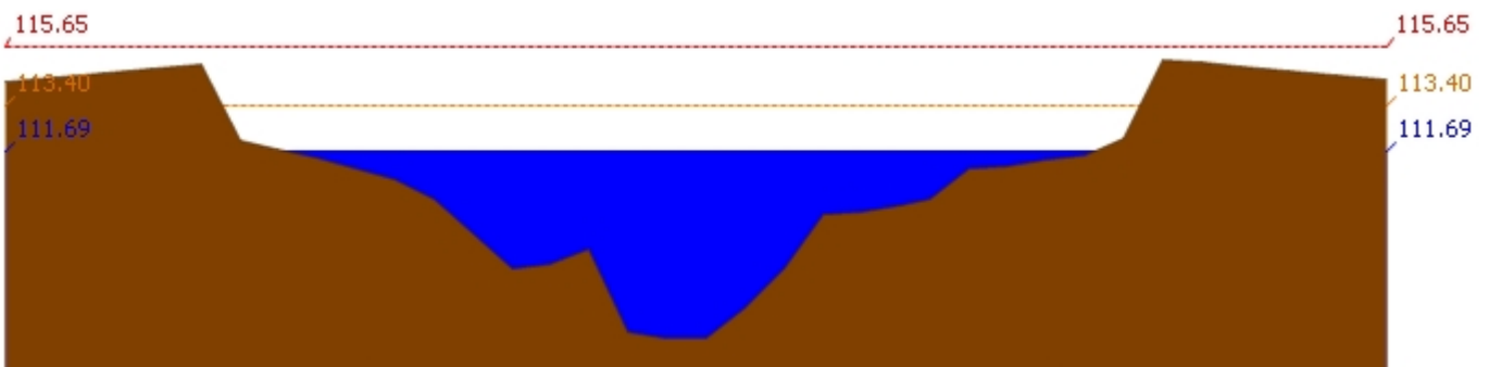
สถานี 120107T แม่น้ำป่าสักที่ อ.เมืองเพชรบูรณ์ ต.นาป่า อ.เมือง จ.เพชรบูรณ์ ระดับน้ำ 111.69 ม.รทก.
