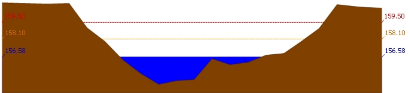
สถานี 120305T ฝายน้ำล้นที่ อ.หล่มเก่า ต.หล่มเก่า อ.หล่มเก่า จ.เพชรบูรณ์ ระดับน้ำ 156.58 ม.รทก.
