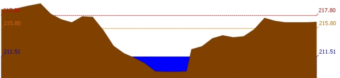
สถานี 120205T แม่น้ำป่าสักที่บ้านอุมกะทาด ต.ศิลา อ.หล่มเก่า จ.เพชรบูรณ์ ระดับน้ำ 211.51 ม.รทก.
