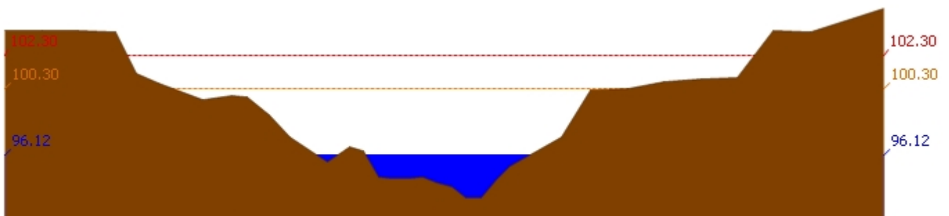
สถานี 120112T แม่น้ำป่าสักที่บ้านหนองแหวน ต.วังมะข่อ อ.เมือง จ.เพชรบูรณ์ ระดับน้ำ 96.12 ม.รทก.
