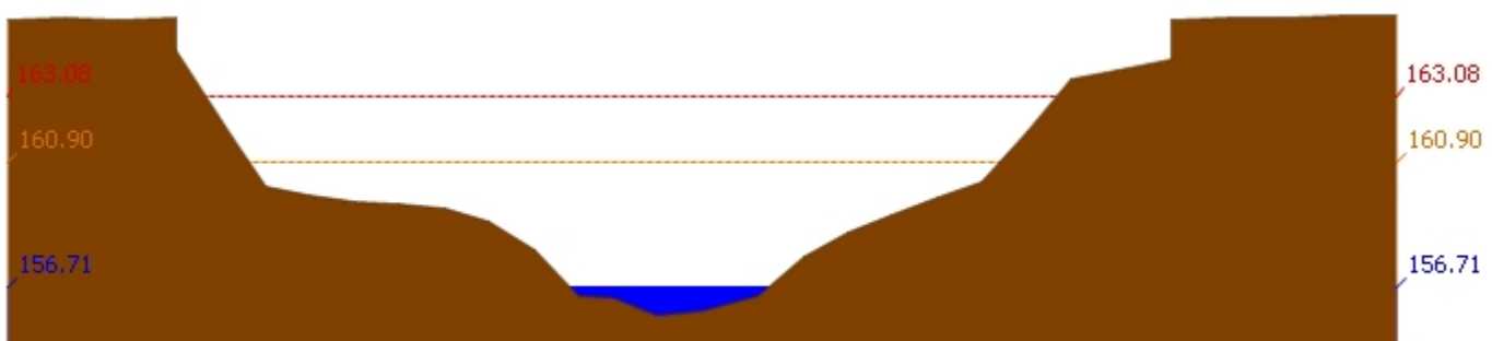
สถานี 120105T แม่น้ำป่าสักที่บ้านวังมลเหนือ ต.ท่าอิฐ อ.หล่มสัก จ.เพชรบูรณ์ ระดับน้ำ 156.71 ม.รทก.
