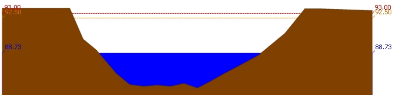
สถานี 120110T แม่น้ำป่าสักที่บ้านวังโบสถ์ ต.วังโบสถ์ อ.หนองไผ่ จ.เพชรบูรณ์ ระดับน้ำ 88.73 ม.รทก.
