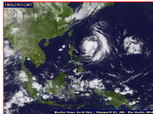
ภาพถ่ายจากดาวเทียม วันที่ 1 ก.ค. 2561
