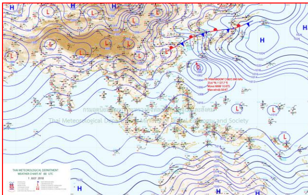
แผนที่อากาศ วันที่ 1 ก.ค. 2561 เวลา 07.00 น.
