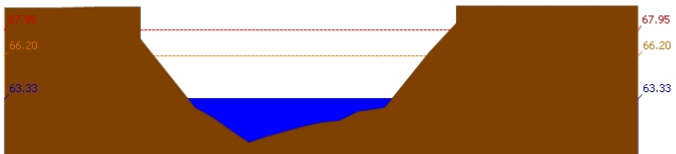
สถานี 110501T น้ำแมวกกที่บ้านคลองสาลี ต.ลาดยาว อ.ลาดยาว จ.นครสวรรค์ ระดับน้ำ 63.33 ม.รทก.
