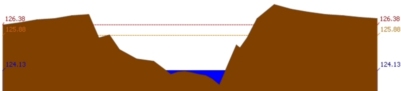
สถานี 110301T คลองโพธิ์ที่บ้านคลองบัวสามัคคี ต.ปางสวรรค์ อ.ชุมตาบง จ.นครสวรรค์ ระดับน้ำ 124.13 ม.รทก.
