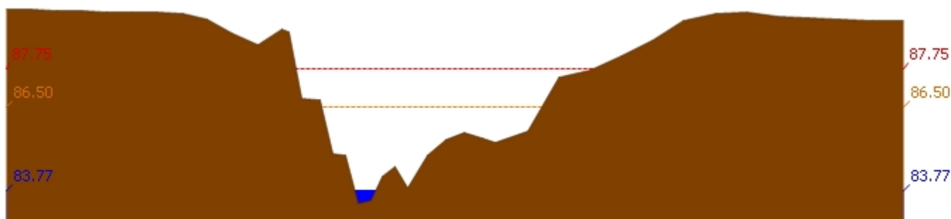
สถานี 110403T ห้วยทับเสลาที่บ้านดินแดง ต.ประดู่ยืน อ.สามโก้ จ.อุทัยธานี ระดับน้ำ 83.77 ม.รทก.
