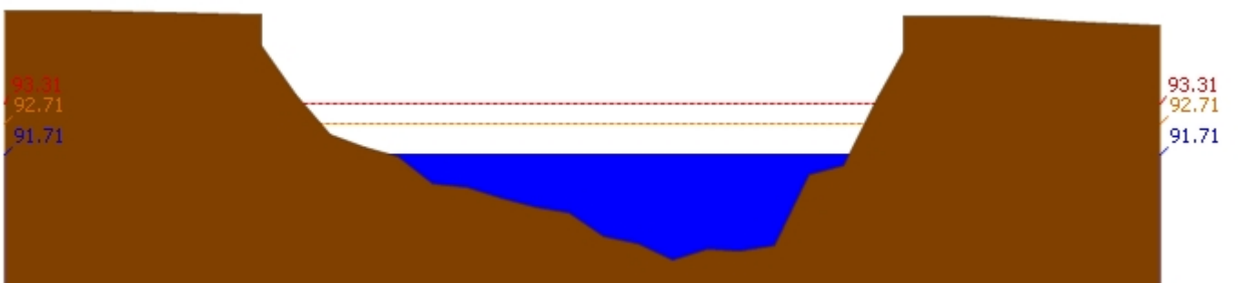
สถานี 061901T คลองแม่ระกาที่บ้านวังชะโอน ต.ท่าไม้ อ.พรานกระต่าย จ.กำแพงเพชร ระดับน้ำ 91.71 ม.รทก.
