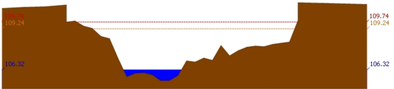
สถานี 061701T ฝายแม่ท้อที่อำเภอเมืองตาก ต.แม่ท้อ อ.เมืองตาก จ.ตาก ระดับน้ำ 106.32 ม.รทก.
