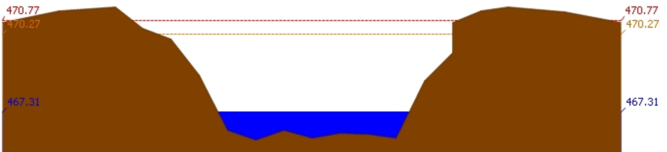
สถานี 061206T น้ำแม่แจ่มที่บ้านทัพ ต.ท่าผา อ.แม่แจ่ม จ.เชียงใหม่ ระดับน้ำ 467.31 ม.รทก.
