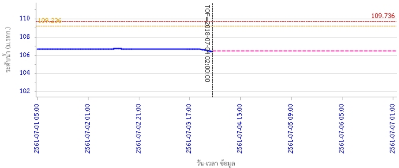
ผลการคำนวณระดับน้ำ สถานี 061801T คลองวังเจ้าที่บ้านคลองลึก ต.เชียงทอง อ.วังเจ้า จ.ตาก
