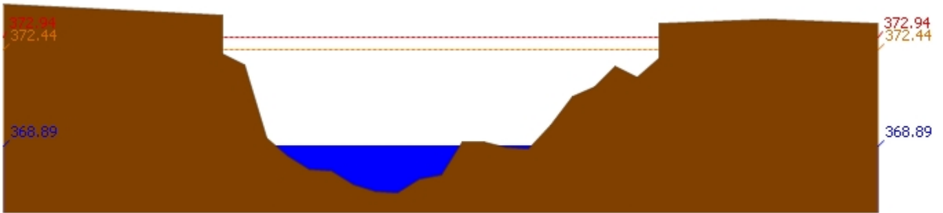
สถานี 060109T แม่ น้ำปิงที่บ้านสบอ้อ ต.แม่ระ อ.เชียงดาว จ.เชียงใหม่ ระดับน้ำ 368.89 ม.รทก.
