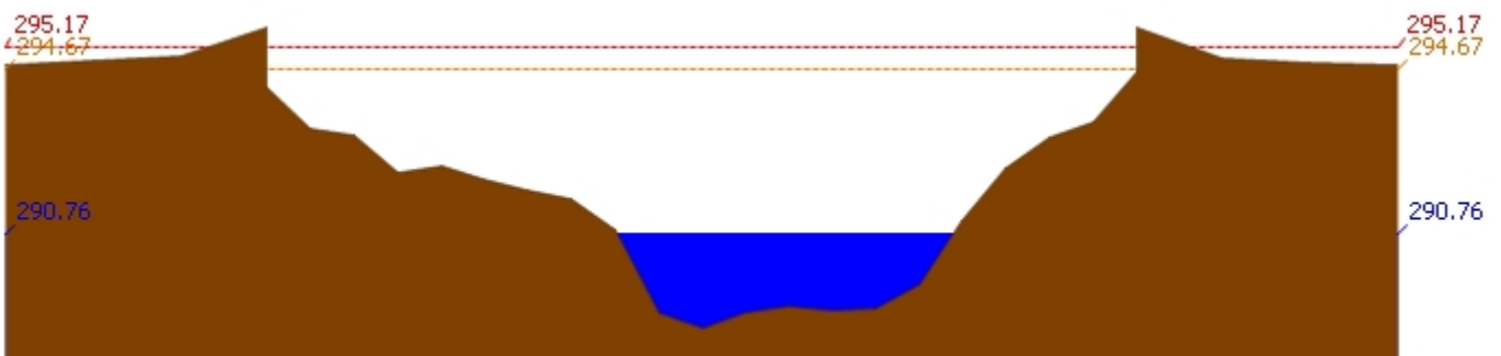
สถานี 060709T น้ำแม่กวางที่ลำพูน ต.เวียงของ อ.เมือง จ.ลำพูน ระดับน้ำ 290.76 ม.รทก.
