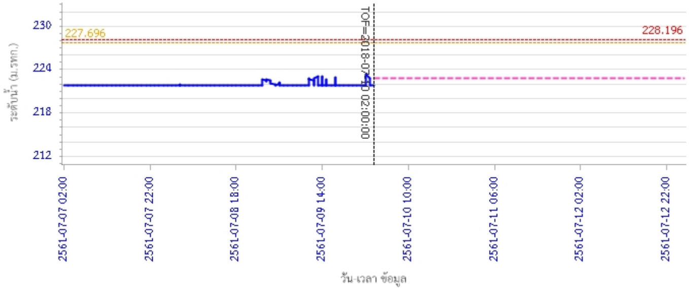
ผลการคำนวณระดับน้ำ สถานี 070115T น้ำแม่วังที่บ้านอ้อ ต.แม่กัวะ อ.สบปราบ จ.ลำปาง
