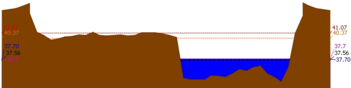
▲ ระดับปัจจุบัน --- ระดับวิกฤติ --- ระดับเฝ้าระวัง ---- เมื่อกาน 7:00 น. - - - - - คาดการณ์ล่วงหน้า 1 วัน สถานี 060110T แม่น้ำปิงที่บ้านบางแก้ว ต.บางแก้ว อ.บรรพตพิสัย จ.นครสวรรค์ ระดับน้ำ 37.70 ม.รทก.
