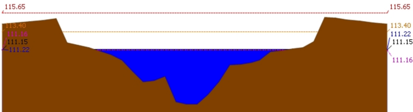
▲ ระดับปัจจุบัน --- ระดับวิกฤติ --- ระดับเฟิาระวัง ---- เมื่อกวาน 7:00 น. - - - - คาคตการลลวงหน้า 1 วัน สถานี 120107T แม่น้ำป่าสักที่ อ.เมืองเพชรบูรณ์ ต.นาป่า อ.เมือง จ.เพชรบูรณ์ ระดับน้ำ 111.22 ม.รทก.
