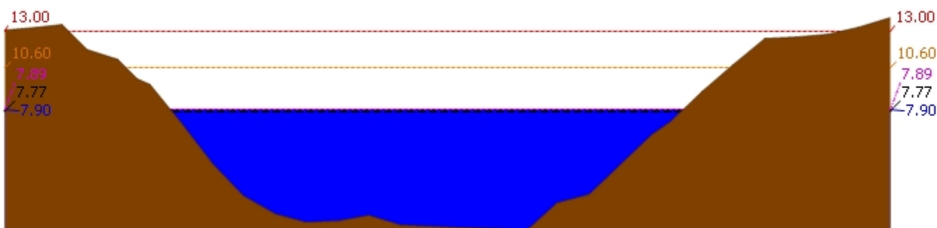
▲ ระดับปัจจุบัน --- ระดับวิกฤติ --- ระดับเฟิาระวัง ---- เมื่อกวาน 7:00 น. - - - - คาคตการลลวงหน้า 1 วัน สถานี 120106T แม่น้ำป่าสักที่ อ.เสาไห้ ต.ศาลาริไทย อ.เสาไห้ จ.สระบุรี ระดับน้ำ 7.90 ม.รทก.
