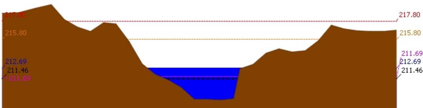
▲ ระดับปัจจุบัน --- ระดับวิกฤติ --- ระดับเฟิาระวัง ---- เมื่อกวาน 7:00 น. - - - - คาคตการลลวงหน้า 1 วัน สถานี 120205T แม่น้ำป่าสักที่ บ้านอุมกะทาด ต.ศิลา อ.หล่มเก่า จ.เพชรบูรณ์ ระดับน้ำ 212.69 ม.รทก.
