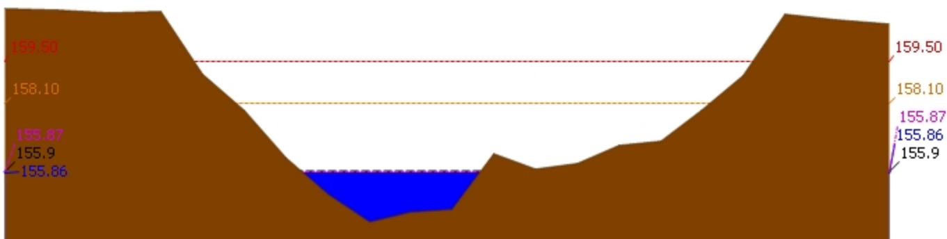
▲ ระดับปัจจุบัน --- ระดับวิกฤติ --- ระดับเฟิาระวัง ---- เมื่อวาน 7:00 น. - - - - - คาดการณ์ล่วงหน้า 1 วัน สถานี 120305T หัวน้ำพุอยู่ที่ อ.หล่มเก่า ต.หล่มเก่า อ.หล่มเก่า จ.เพชรบูรณ์ ระดับน้ำ 155.86 ม.รทก.
