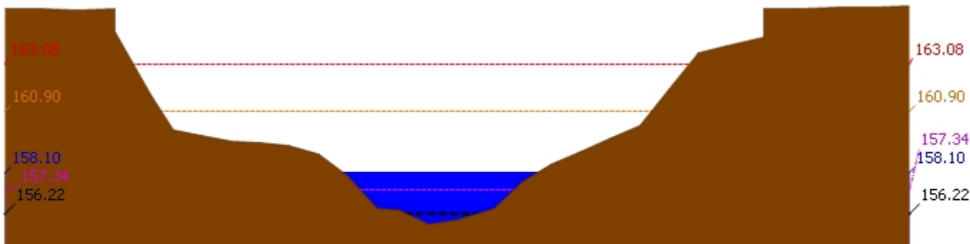
▲ ระดับปัจจุบัน --- ระดับวิกฤติ --- ระดับเฟิาระวัง ---- เมื่อวาน 7:00 น. - - - - - คาดการณ์ล่วงหน้า 1 วัน สถานี 120105T แม่น้ำป่าสักที่บ้านวังมเหนื่อ ต.ท่าอินดู อ.หล่มสัก จ.เพชรบูรณ์ ระดับน้ำ 158.10 ม.รทก.
