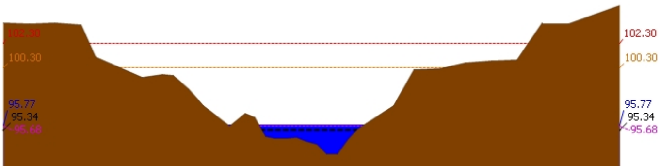
▲ ระดับปัจจุบัน --- ระดับวิกฤติ --- ระดับเฟิาระวัง ---- เมื่อวาน 7:00 น. - - - - - คาดการณ์ล่วงหน้า 1 วัน สถานี 120112T แม่น้ำป่าสักที่บ้านหนองแหวน ต.วังมะข่อ อ.เมือง จ.เพชรบูรณ์ ระดับน้ำ 95.77 ม.รทก.
