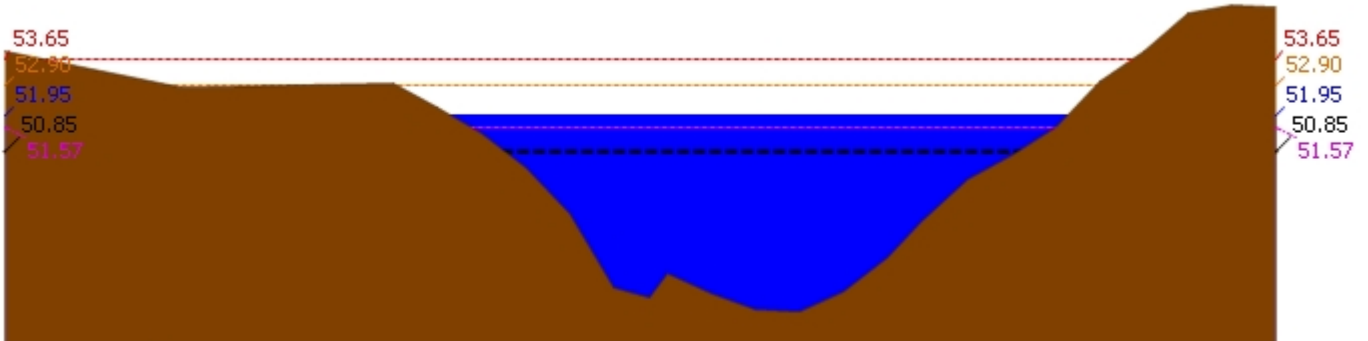
▲ ระดับปัจจุบัน --- ระดับวิกฤติ --- ระดับฝายระวัง ----- เมื่อวาน 7:00 น. - - - - - คาดการณ์ล่วงหน้า 1 วัน สถานี 120113T แม่น้ำป่าสักที่บ้านเขาค้าง ต.คลองกระจิง อ.ศรีเทพ จ.เพชรบูรณ์ ระดับน้ำ 51.95 ม.รทก.
