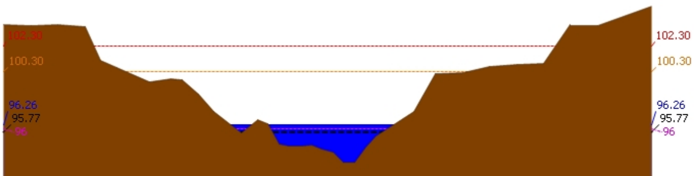
▲ ระดับปัจจุบัน --- ระดับวิกฤติ --- ระดับเฟิาระวัง ---- เมื่อกวาน 7:00 น. - - - - - คาดการณ์ล่วงหน้า 1 วัน สถานี 120112T แม่น้ำป่าสักที่บ้านหนองแหวน ต.วังมะซ่อ อ.เมือง จ.เพชรบูรณ์ ระดับน้ำ 96.26 ม.รทก.
