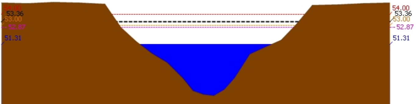
▲ ระดับปัจจุบัน --- ระดับวิกฤติ --- ระดับฝายระวัง ----- เมื่อวาน 7:00 น. - - - - - คาดการณ์ล่วงหน้า 1 วัน สถานี 120702T ลำสนธิที่บ้านท่าช้าง ต.หนองขาหย่าง อ.ชัยบาดาล จ.ลพบุรี ระดับน้ำ 51.31 ม.รทก.
