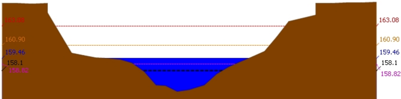
▲ ระดับปัจจุบัน --- ระดับวิกฤติ --- ระดับเฟิาระวัง ---- เมื่อกวาน 7:00 น. - - - - - คาดการณ์ล่วงหน้า 1 วัน สถานี 120105T แม่น้ำป่าสักที่บ้านวังมเสหนือ ต.ทำอึบุญ อ.หล่มสัก จ.เพชรบูรณ์ ระดับน้ำ 159.46 ม.รทก.
