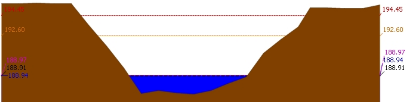
▲ ระดับปัจจุบัน --- ระดับวิกฤติ --- ระดับฝายระวัง ----- เมื่อวาน 7:00 น. - - - - - คาดการณ์ล่วงหน้า 1 วัน สถานี 120901T ห้วยมวกเหล็กที่ อ.มวกเหล็ก ต.มวกเหล็ก อ.มวกเหล็ก จ.สระบุรี ระดับน้ำ 188.94 ม.รทก.
