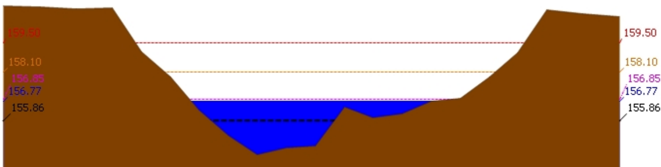
▲ ระดับปัจจุบัน --- ระดับวิกฤติ --- ระดับเฟิาระวัง ---- เมื่อกวาน 7:00 น. - - - - - คาดการณ์ล่วงหน้า 1 วัน สถานี 120305T หัวน้ำพุทที่ อ.หล่มเก่า ต.หล่มเก่า อ.หล่มเก่า จ.เพชรบูรณ์ ระดับน้ำ 156.77 ม.รทก.
