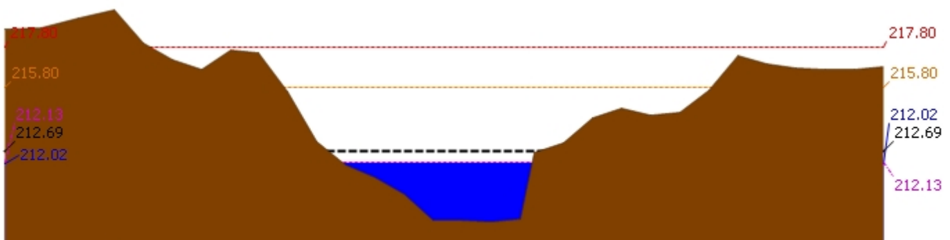
▲ ระดับปัจจุบัน --- ระดับวิกฤติ --- ระดับฝายระวัง ---- เมื่อกวาน 7:00 น. - - - - - คาดการณ์ล่วงหน้า 1 วัน สถานี 120205T แม่น้ำป่าสักที่ บ้านอุมกะทาด ต.ศิลา อ.หล่มเก่า จ.เพชรบูรณ์ ระดับน้ำ 212.02 ม.รทก.
