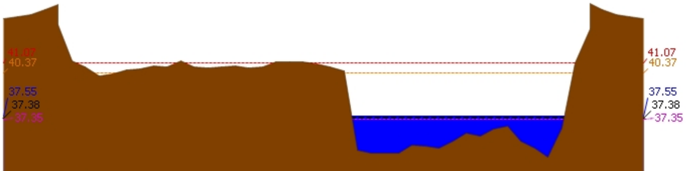
▲ ระดับปัจจุบัน --- ระดับวิกฤติ --- ระดับเฝ้าระวัง ---- เมื่อวาน 7:00 น. - - - - - คาดการณ์ล่วงหน้า 1 วัน สถานี 060110T แม่น้ำปิงที่บ้านบางแก้ว ต.บางแก้ว อ.บรรพตพิสัย จ.นครสวรรค์ ระดับน้ำ 37.55 ม.รทก.
