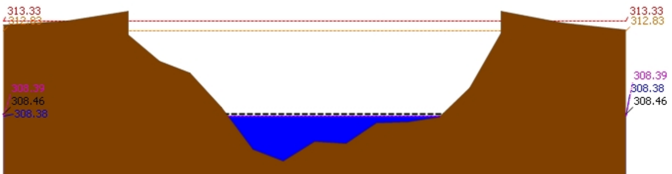
▲ ระดับปัจจุบัน --- ระดับวิกฤติ --- ระดับเฝ้าระวัง ---- เมื่อวาน 7:00 น. - - - - - คาดการณ์ล่วงหน้า 1 วัน สถานี 060814T น้ำแม่ฆานที่บ้านท่าโป่ง ต.บ้านแม อ.สันป่าตอง จ.เชียงใหม่ ระดับน้ำ 308.38 ม.รทก.
