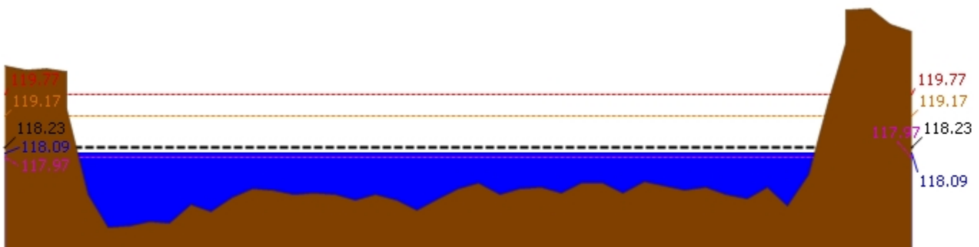
▲ ระดับปัจจุบัน --- ระดับวิกฤติ --- ระดับเฝ้าระวัง ---- เมื่อวาน 7:00 น. - - - - - คาดการณ์ล่วงหน้า 1 วัน สถานี 060111T แม่น้ำปิงที่บ้านปากร่องห้วยจี่ ต.ตากออก อ.บ้านตาก จ.ตาก ระดับน้ำ 118.09 ม.รทก.
