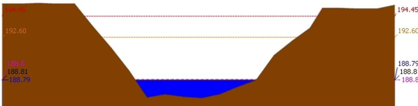
▲ ระดับปัจจุบัน --- ระดับวิกฤติ --- ระดับฝายระวัง ---- เมื่อวาน 7:00 น. - - - - - คาดการณ์ล่วงหน้า 1 วัน สถานี 120901T ห้วยมวกเหล็กที่ อ.มวกเหล็ก ต.มวกเหล็ก อ.มวกเหล็ก จ.สระบุรี ระดับน้ำ 188.79 ม.รทก.
