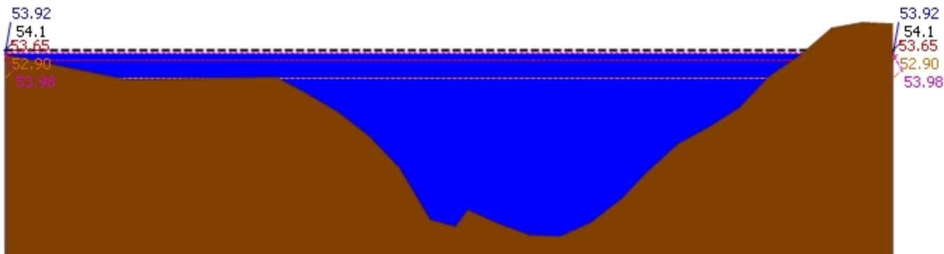
▲ ระดับปัจจุบัน --- ระดับวิกฤติ --- ระดับฝายระวัง ---- เมื่อวาน 7:00 น. - - - - - คาดการณ์ล่วงหน้า 1 วัน สถานี 120113T แม่น้ำป่าสักที่บ้านเขาค้าง ต.คลองกระจิง อ.ศรีเทพ จ.เพชรบูรณ์ ระดับน้ำ 53.92 ม.รทก.
