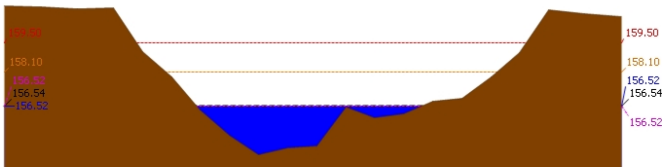
▲ ระดับปัจจุบัน --- ระดับวิกฤติ --- ระดับเฝ้าระวัง ---- เมื่อวาน 7:00 น. - - - - - คาดการณ์ล่วงหน้า 1 วัน สถานี 120305T หัวน้ำพุที่ อ.หล่มเก่า ต.หล่มเก่า อ.หล่มเก่า จ.เพชรบูรณ์ ระดับน้ำ 156.52 ม.รทก.
