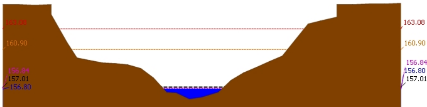
▲ ระดับปัจจุบัน --- ระดับวิกฤติ --- ระดับเฝ้าระวัง ---- เมื่อวาน 7:00 น. - - - - - คาดการณ์ล่วงหน้า 1 วัน สถานี 120105T แม่น้ำป่าสักที่บ้านวังมเสหนือ ต.ทำอัญญ อ.หล่มสัก จ.เพชรบูรณ์ ระดับน้ำ 156.80 ม.รทก.
