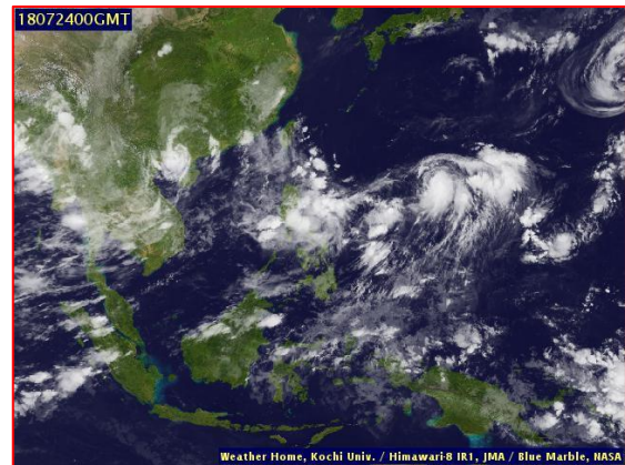
ภาพถ่ายจากดาวเทียม วันที่ 24 ก.ค. 2561 เวลา 07.00 น.
