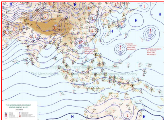
แผนที่อากาศวันที่ 24 ก.ค. 2561 เวลา 07.00 น.
