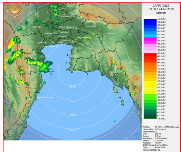
ภาพเรดาร์ตรวจอากาศ “สถานีสัตหีบ” ณ วันที่ 24 กรกฎาคม 2561 เวลา 10.00 น. (ที่มา : กรมอุตุนิยมวิทยา)
