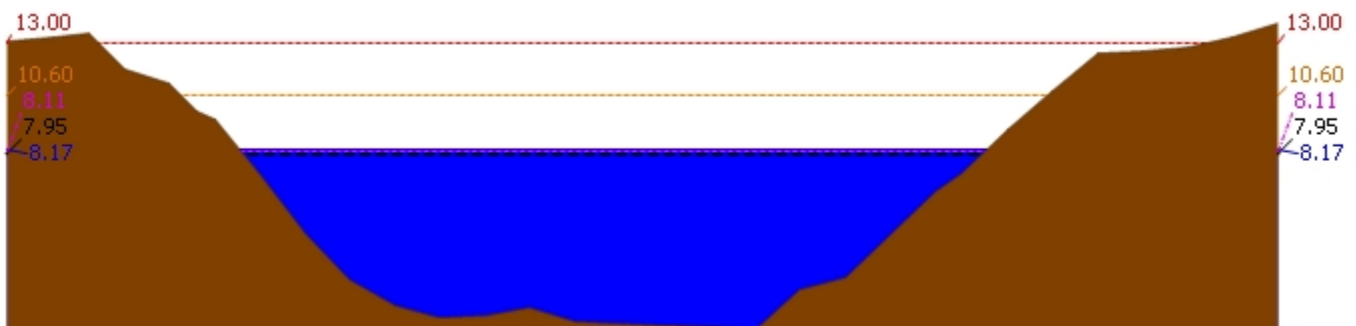
▲ ระดับปัจจุบัน --- ระดับวิกฤติ --- ระดับเฟิาระวัง ---- เมือวาน 7:00 น. - - - - คาคการลลวงหน้า 1 วัน สถานี 120106T แม่น้ำป่าสักที่ อ.เสาไห้ ต.ศาลาริไทย อ.เสาไห้ จ.สระบุรี ระดับน้ำ 8.17 ม.รทก.
