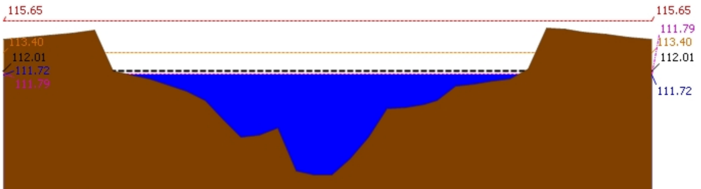
▲ ระดับปัจจุบัน --- ระดับวิกฤติ --- ระดับเฟิาระวัง ---- เมือวาน 7:00 น. - - - - คาคการลลวงหน้า 1 วัน สถานี 120107T แม่น้ำป่าสักที่ อ.เมืองเพชรบูรณ์ ต.นาป่า อ.เมือง จ.เพชรบูรณ์ ระดับน้ำ 111.72 ม.รทก.
