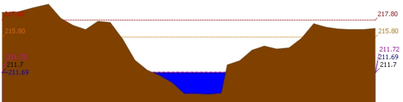
▲ ระดับปัจจุบัน --- ระดับวิกฤติ --- ระดับเฟิาระวัง ---- เมือวาน 7:00 น. - - - - คาคการลลวงหน้า 1 วัน สถานี 120205T แม่น้ำป่าสักที่ บ้านอุมกะทาด ต.ศิลา อ.หล่มเก่า จ.เพชรบูรณ์ ระดับน้ำ 211.69 ม.รทก.
