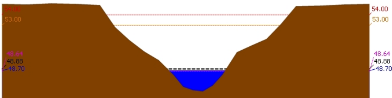
▲ ระดับปัจจุบัน --- ระดับวิกฤติ --- ระดับฝายระวัง ---- เมื่อวาน 7:00 น. - - - - - คาดการณ์ล่วงหน้า 1 วัน สถานี 120702T ลำสนธิที่บ้านท่าช้าง ต.หนองขาหย่าง อ.ชัยบาดาล จ.ลพบุรี ระดับน้ำ 48.70 ม.รทก.
