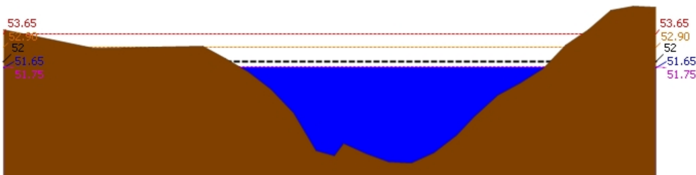
▲ ระดับปัจจุบัน --- ระดับวิกฤติ --- ระดับฝายระวัง ---- เมื่อวาน 7:00 น. - - - - - คาดการณ์ล่วงหน้า 1 วัน สถานี 120113T แม่น้ำป่าสักที่บ้านเขาค้าง ต.คลองกระจิง อ.ศรีเทพ จ.เพชรบูรณ์ ระดับน้ำ 51.65 ม.รทก.
