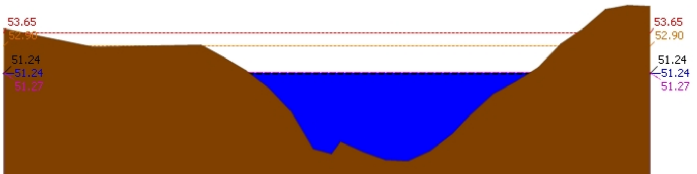
▲ ระดับปัจจุบัน --- ระดับวิกฤติ --- ระดับเฝ้าระวัง - - - - - เมื่อวาน 7:00 น. - - - - - คาดการณ์ล่วงหน้า 1 วัน สถานี 120113T แม่น้ำป่าสักที่บ้านเขาค้าง ต.คลองกระจิง อ.ศรีเทพ จ.เพชรบูรณ์ ระดับน้ำ 51.24 ม.รทก.
