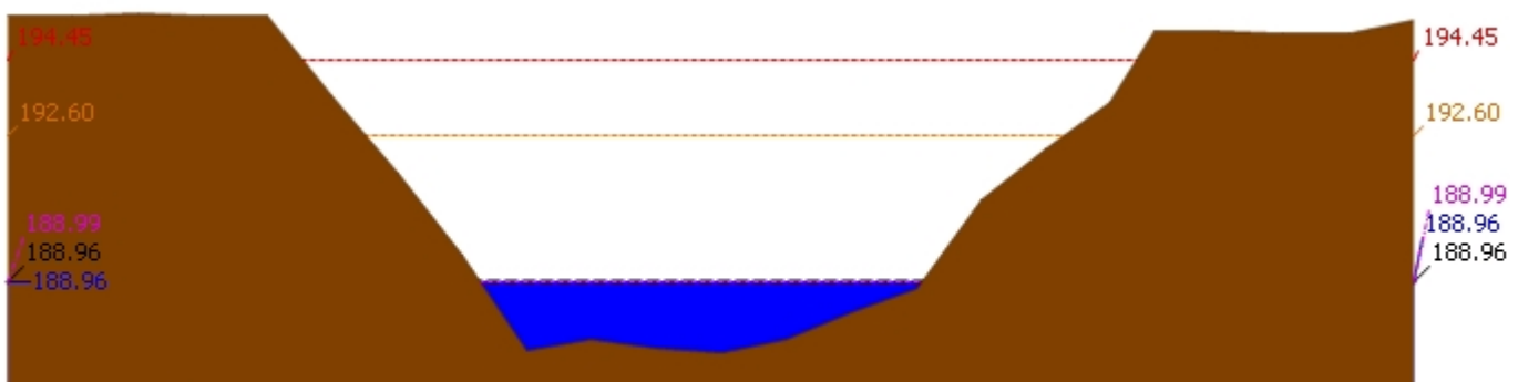
▲ ระดับปัจจุบัน --- ระดับวิกฤติ --- ระดับเฝ้าระวัง - - - - - เมื่อวาน 7:00 น. - - - - - คาดการณ์ล่วงหน้า 1 วัน สถานี 120901T ห้วยมวกเหล็กที่ อ.มวกเหล็ก ต.มวกเหล็ก อ.มวกเหล็ก จ.สระบุรี ระดับน้ำ 188.96 ม.รทก.
