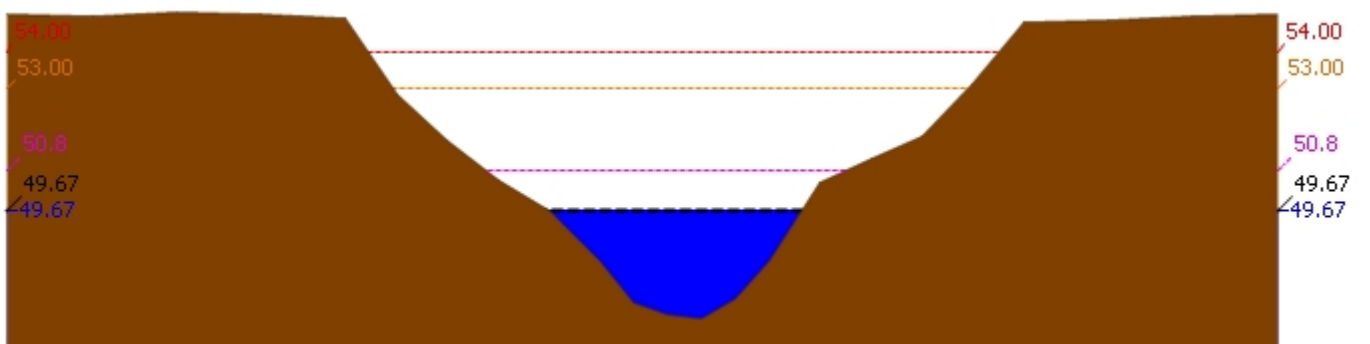
▲ ระดับปัจจุบัน --- ระดับวิกฤติ --- ระดับเฝ้าระวัง - - - - - เมื่อวาน 7:00 น. - - - - - คาดการณ์ล่วงหน้า 1 วัน สถานี 120702T ลำสนธิที่บ้านท่าช้าง ต.หนองขาหย่าง อ.ชัยบาดาล จ.ลพบุรี ระดับน้ำ 49.67 ม.รทก.
