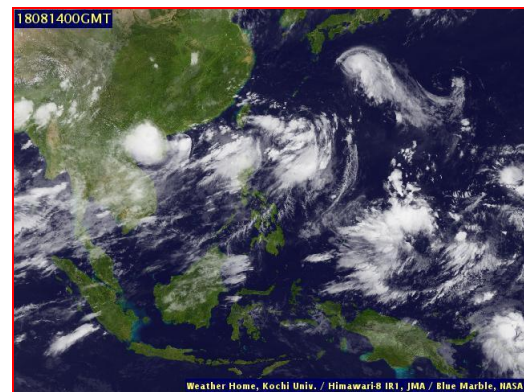
ภาพถ่ายจากดาวเทียม วันที่ 14 ส.ค. 2561
