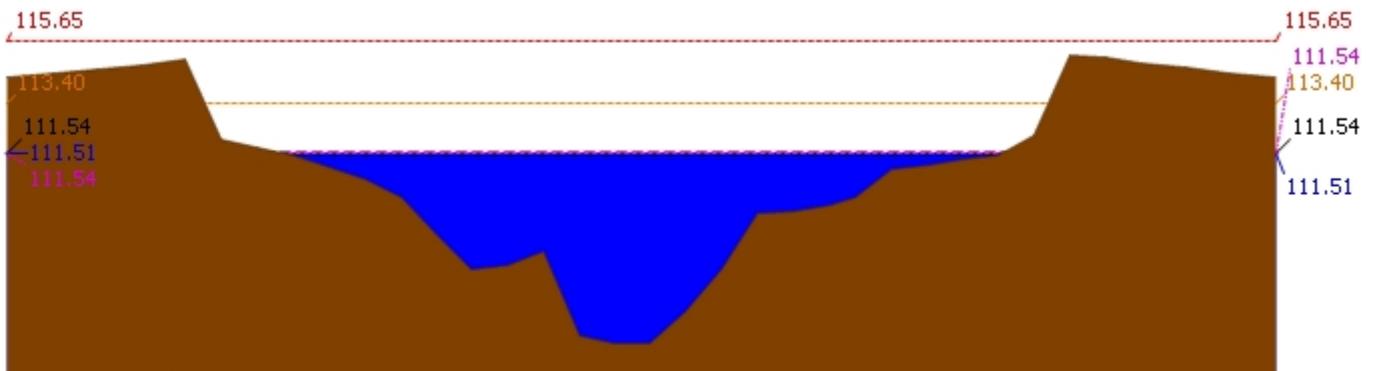
▲ ระดับปัจจุบัน --- ระดับวิกฤติ --- ระดับฝักระวัง ---- เมื่อกวาน 7:00 น. - - - - คาดการณ์ล่วงหน้า 1 วัน สถานี 120107T แม่น้ำป่าสักที่ อ.เมืองเพชรบูรณ์ ต.นาป่า อ.เมือง จ.เพชรบูรณ์ ระดับน้ำ 111.51 ม.รทก.
