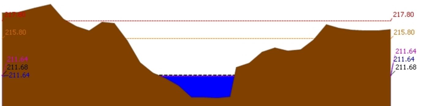
▲ ระดับปัจจุบัน --- ระดับวิกฤติ --- ระดับฝักระวัง ---- เมื่อกวาน 7:00 น. - - - - คาดการณ์ล่วงหน้า 1 วัน สถานี 120205T แม่น้ำป่าสักที่บ้านอุมกะทาด ต.ศิลา อ.หล่มเก่า จ.เพชรบูรณ์ ระดับน้ำ 211.64 ม.รทก.
