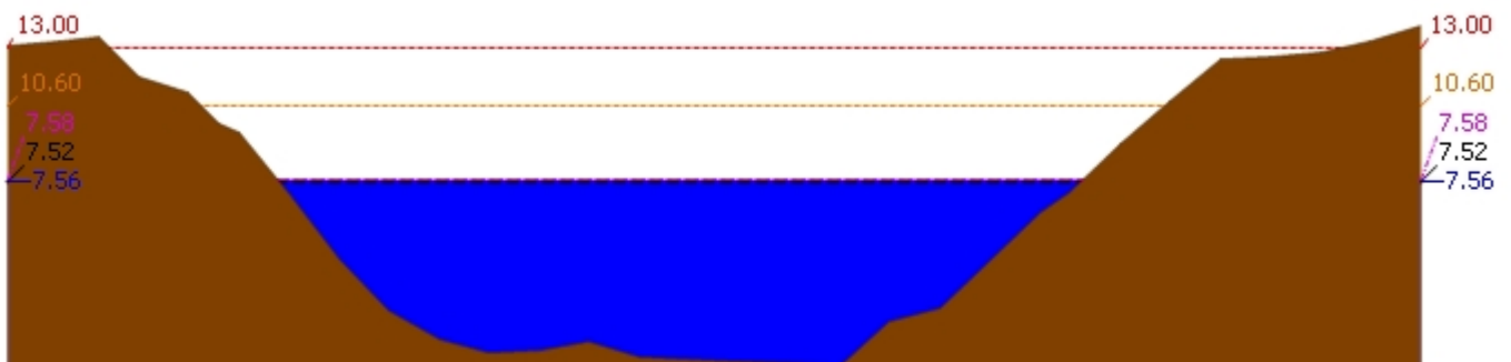
▲ ระดับปัจจุบัน --- ระดับวิกฤติ --- ระดับฝักระวัง ---- เมื่อกวาน 7:00 น. - - - - คาดการณ์ล่วงหน้า 1 วัน สถานี 120106T แม่น้ำป่าสักที่ อ.เสาไห้ ต.ศาลารีย์ไทย อ.เสาไห้ จ.สระบุรี ระดับน้ำ 7.56 ม.รทก.
