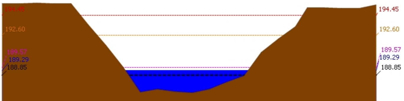
▲ ระดับปัจจุบัน --- ระดับวิกฤติ --- ระดับเฝ้าระวัง ---- เมื่อกว่า 7:00 น. - - - - - คาดการณ์ล่วงหน้า 1 วัน สถานี 120901T ห้วยมวกเหล็กที่ อ.มวกเหล็ก ต.มวกเหล็ก อ.มวกเหล็ก จ.สระบุรี ระดับน้ำ 189.29 ม.รทก.
