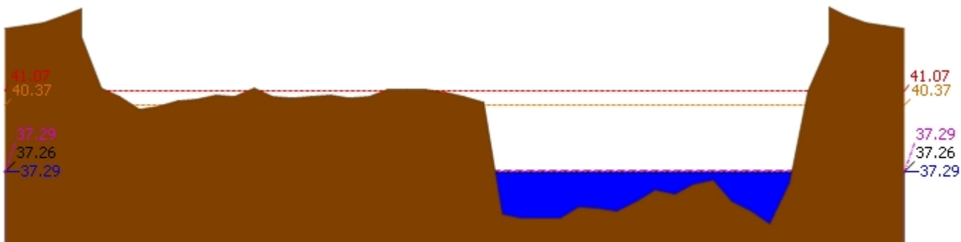
▲ ระดับปัจจุบัน --- ระดับวิกฤติ --- ระดับเฝ้าระวัง ---- เมื่อวาน 7:00 น. - - - - คาดการณ์ล่วงหน้า 1 วัน สถานี 060110T แม่น้ำปิงที่บ้านบางแก้ว ต.บางแก้ว อ.บรรพตพิสัย จ.นครสวรรค์ ระดับน้ำ 37.29 ม.รทก.
