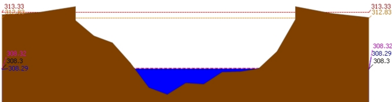
▲ ระดับปัจจุบัน --- ระดับวิกฤติ --- ระดับเฝ้าระวัง ---- เมื่อวาน 7:00 น. - - - - คาดการณ์ล่วงหน้า 1 วัน สถานี 060814T น้ำแม่ขานที่บ้านท่าโป่ง ต.บ้านแม่ อ.สันป่าตอง จ.เชียงใหม่ ระดับน้ำ 308.29 ม.รทก.
