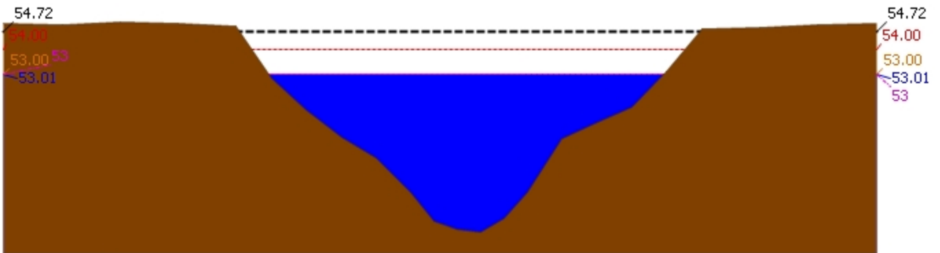
▲ ระดับปัจจุบัน --- ระดับวิกฤติ --- ระดับฝายระวัง ---- เมื่อวาน 7:00 น. - - - - - คาดการณ์ล่วงหน้า 1 วัน สถานี 120702T ลำสนธิที่บ้านท่าช้าง ต.หนองขาหย่าง อ.ชัยบาดาล จ.ลพบุรี ระดับน้ำ 53.01 ม.รทก.
