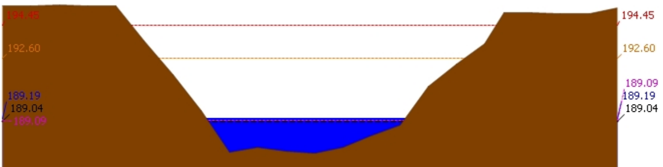
▲ ระดับปัจจุบัน --- ระดับวิกฤติ --- ระดับฝายระวัง ---- เมื่อวาน 7:00 น. - - - - - คาดการณ์ล่วงหน้า 1 วัน สถานี 120901T ห้วยมวกเหล็กที่ อ.มวกเหล็ก ต.มวกเหล็ก อ.มวกเหล็ก จ.สระบุรี ระดับน้ำ 189.19 ม.รทก.
