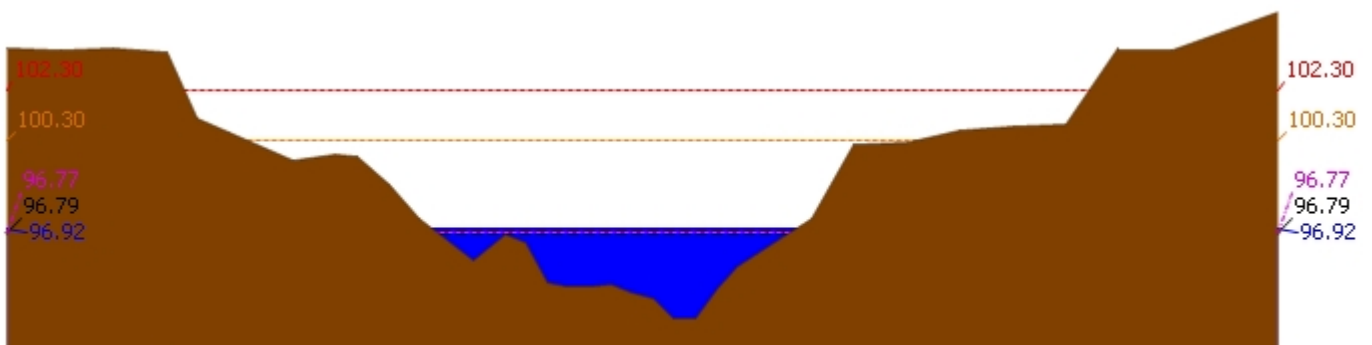
▲ ระดับปัจจุบัน --- ระดับวิกฤติ --- ระดับฝายระวัง ---- เมื่อวาน 7:00 น. - - - - คาดการณ์ล่วงหน้า 1 วัน สถานี 120112T แม่น้ำป่าสักที่บ้านหนองแหวน ต.วังมะข่อ อ.เมือง จ.เพชรบูรณ์ ระดับน้ำ 96.92 ม.รทก.
