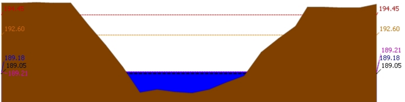
▲ ระดับปัจจุบัน --- ระดับวิกฤติ --- ระดับเฝ้าระวัง ---- เมื่อกาน 7:00 น. - - - - - คาดการณ์ล่วงหน้า 1 วัน สถานี 120901T ห้วยมวกเหล็กที่ อ.มวกเหล็ก ต.มวกเหล็ก อ.มวกเหล็ก จ.สระบุรี ระดับน้ำ 189.18 ม.รทก.
