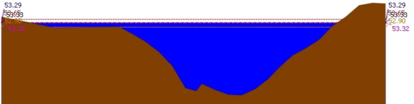
▲ ระดับปัจจุบัน --- ระดับวิกฤติ --- ระดับเฝ้าระวัง ---- เมื่อกาน 7:00 น. - - - - - คาดการณ์ล่วงหน้า 1 วัน สถานี 120113T แม่น้ำป่าสักที่บ้านเขาค้าง ต.คลองกระจิง อ.ศรีเทพ จ.เพชรบูรณ์ ระดับน้ำ 53.29 ม.รทก.
