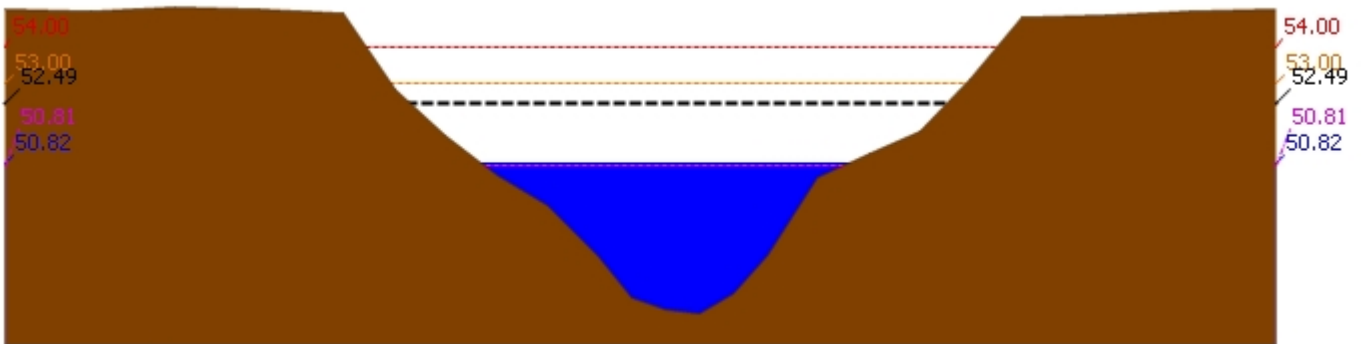
▲ ระดับปัจจุบัน --- ระดับวิกฤติ --- ระดับเฝ้าระวัง ---- เมื่อกาน 7:00 น. - - - - - คาดการณ์ล่วงหน้า 1 วัน สถานี 120702T ลำสนธิที่บ้านท่าช้าง ต.หนองขาหย่าง อ.ชัยบาดาล จ.ลพบุรี ระดับน้ำ 50.82 ม.รทก.
