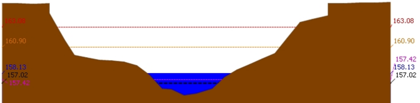
▲ ระดับปัจจุบัน --- ระดับวิกฤติ --- ระดับฝายระวัง ---- เมื่อวาน 7:00 น. - - - - คาดการณ์ล่วงหน้า 1 วัน สถานี 120105T แม่น้ำป่าสักที่บ้านวังมเสหนือ ต.ทำอัญญ อ.หล่มสัก จ.เพชรบูรณ์ ระดับน้ำ 158.13 ม.รทก.
