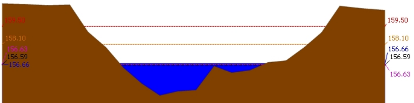
▲ ระดับปัจจุบัน --- ระดับวิกฤติ --- ระดับฝายระวัง ---- เมื่อวาน 7:00 น. - - - - คาดการณ์ล่วงหน้า 1 วัน สถานี 120305T หัวน้ำพุอยู่ที่ อ.หล่มเก่า ต.หล่มเก่า อ.หล่มเก่า จ.เพชรบูรณ์ ระดับน้ำ 156.66 ม.รทก.
