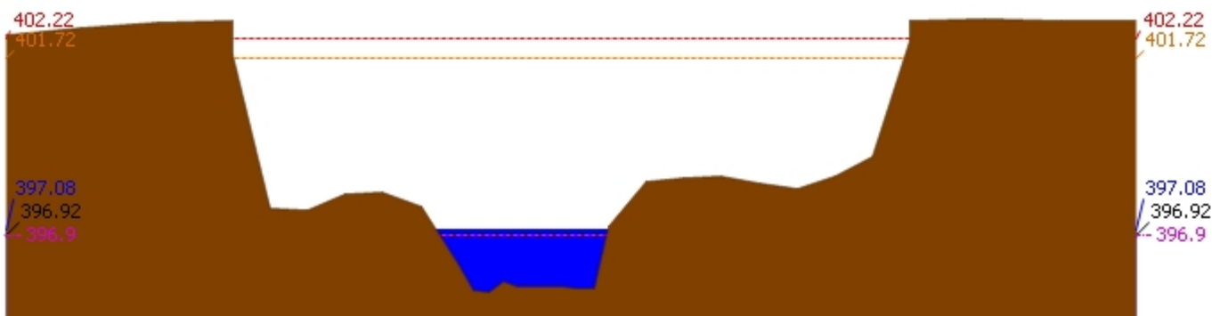
สถานี 060305T น้ำแม่จัดที่บ้านโป่งบัวบาน ต.แม่ปิ้ง อ.พร้าว จ.เชียงใหม่ ระดับน้ำ 397.08 ม.รทก.
