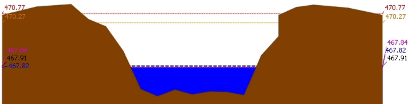
สถานี 061206T น้ำแม่แจ่มที่บ้านทัพ ต.ท่าผา อ.แม่แจ่ม จ.เชียงใหม่ ระดับน้ำ 467.82 ม.รทก.
