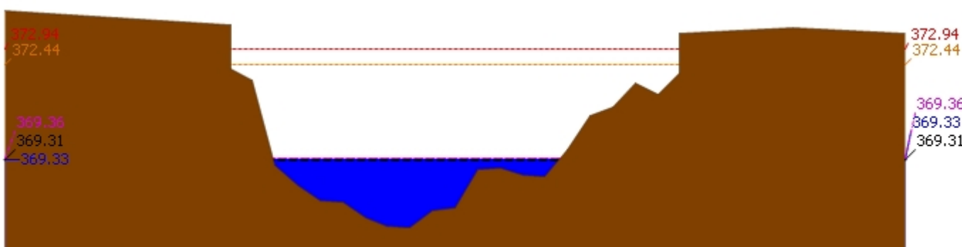
สถานี 060109T แม่น้ำปิงที่บ้านสบอ้อ ต.แม่บะ อ.เชียงดาว จ.เชียงใหม่ ระดับน้ำ 369.33 ม.รทก.
