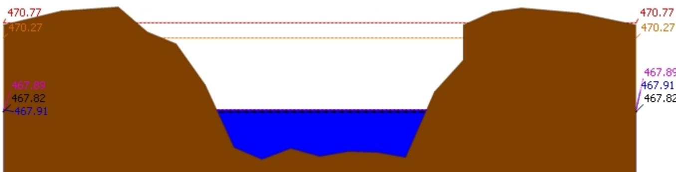
สถานี 061206T น้ำแม่แจ่มที่บ้านทัพ ต.ท่าผา อ.แม่แจ่ม จ.เชียงใหม่ ระดับน้ำ 467.91 ม.รทก.
