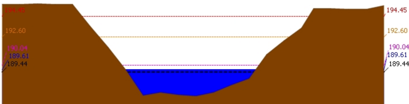
▲ ระดับปัจจุบัน --- ระดับวิกฤติ --- ระดับเฝ้าระวัง ---- เมื่อวาน 7:00 น. - - - - คาดการณ์ล่วงหน้า 1 วัน สถานี 120901T ห้วยมวกเหล็กที่ อ.มวกเหล็ก ต.มวกเหล็ก อ.มวกเหล็ก จ.สระบุรี ระดับน้ำ 189.61 ม.รทก.
