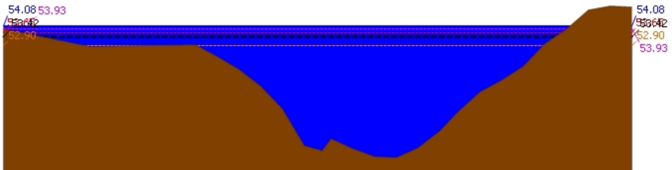
▲ ระดับปัจจุบัน --- ระดับวิกฤติ --- ระดับเฝ้าระวัง ---- เมื่อวาน 7:00 น. - - - - คาดการณ์ล่วงหน้า 1 วัน สถานี 120113T แม่น้ำป่าสักที่บ้านเขาค้าง ต.คลองกระจิง อ.ศรีเทพ จ.เพชรบูรณ์ ระดับน้ำ 54.08 ม.รทก.
