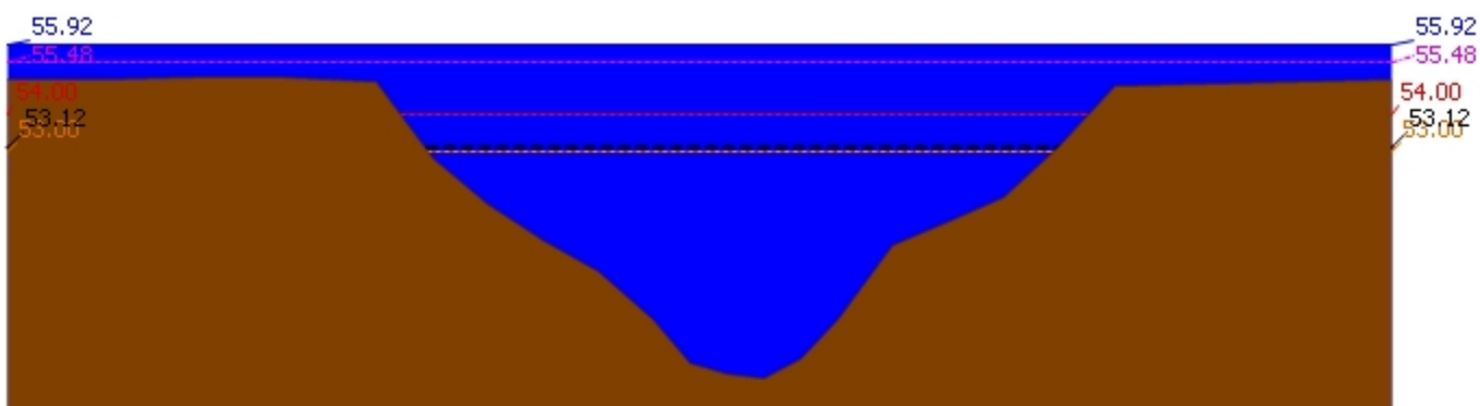
▲ ระดับปัจจุบัน --- ระดับวิกฤติ --- ระดับเฝ้าระวัง ---- เมื่อวาน 7:00 น. - - - - คาดการณ์ล่วงหน้า 1 วัน สถานี 120702T ลำสนธิที่บ้านท่าช้าง ต.หนองขาหย่าง อ.ชัยบาดาล จ.ลพบุรี ระดับน้ำ 55.92 ม.รทก.
