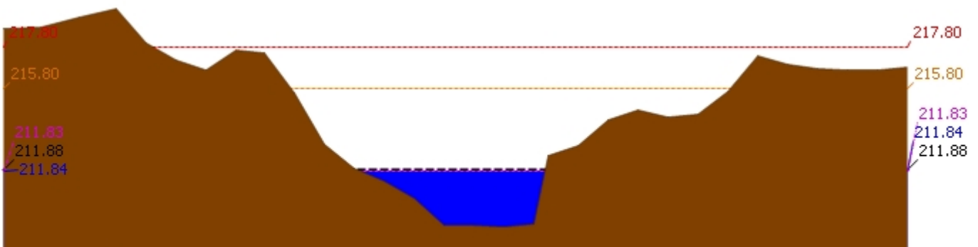
▲ ระดับปัจจุบัน --- ระดับวิกฤติ --- ระดับฝายระวัง ---- เมื่อกวาน 7:00 น. - - - - คาคการล่ลวงหน้า 1 วัน สถานี 120205T แม่น้ำป่าสักที่บ้านอู่กะทาด ต.ศิลา อ.หล่มเก่า จ.เพชรบูรณ์ ระดับน้ำ 211.84 ม.รทก.
