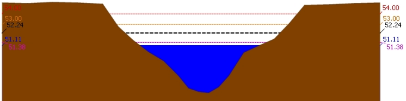
▲ ระดับปัจจุบัน --- ระดับวิกฤติ --- ระดับเฝ้าระวัง ---- เมื่อวาน 7:00 น. - - - - - คาดการณ์ล่วงหน้า 1 วัน สถานี 120702T ลำสนธิที่บ้านท่าช้าง ต.หนองขาหย่าง อ.ชัยบาดาล จ.ลพบุรี ระดับน้ำ 51.11 ม.รทก.
