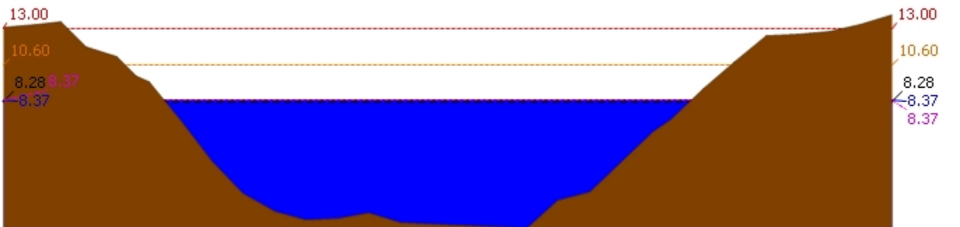
▲ ระดับปัจจุบัน --- ระดับวิกฤติ --- ระดับฝายระวัง ---- เมื่อกวาน 7:00 น. - - - - คาคการล่ลวงหน้า 1 วัน สถานี 120106T แม่น้ำป่าสักที่ อ.เสาไห้ ต.ศาลารี่ไทย อ.เสาไห้ จ.สระบุรี ระดับน้ำ 8.37 ม.รทก.
