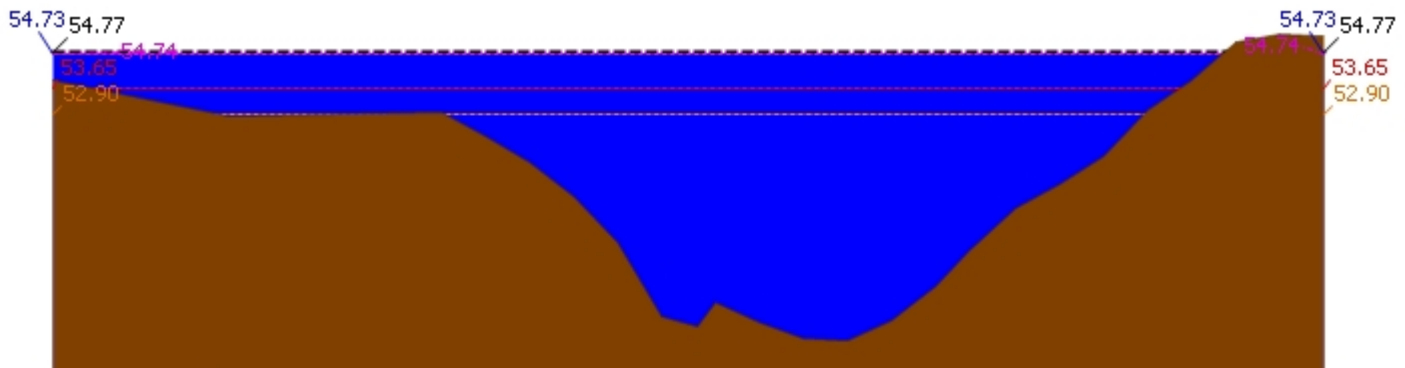
▲ ระดับปัจจุบัน --- ระดับวิกฤติ --- ระดับเฝ้าระวัง ---- เมื่อวาน 7:00 น. - - - - - คาดการณ์ล่วงหน้า 1 วัน สถานี 120113T แม่น้ำป่าสักที่บ้านเขาค้าง ต.คลองกระจิง อ.ศรีเทพ จ.เพชรบูรณ์ ระดับน้ำ 54.73 ม.รทก.
