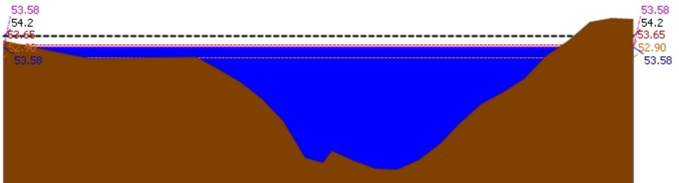
▲ ระดับปัจจุบัน --- ระดับวิกฤติ --- ระดับเฝ้าระวัง ---- เมื่อวาน 7:00 น. - - - - คาดการณ์ล่วงหน้า 1 วัน สถานี 120113T แม่น้ำป่าสักที่บ้านเขาค้าง ต.คลองกระจิง อ.ศรีเทพ จ.เพชรบูรณ์ ระดับน้ำ 53.58 ม.รทก.
