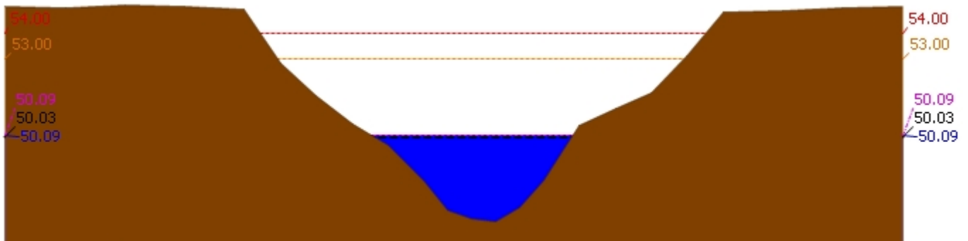
▲ ระดับปัจจุบัน --- ระดับวิกฤติ --- ระดับเฝ้าระวัง ---- เมื่อวาน 7:00 น. - - - - คาดการณ์ล่วงหน้า 1 วัน สถานี 120702T ลำสนธิที่บ้านท่าช้าง ต.หนองขาหย่าง อ.ชัยบาดาล จ.ลพบุรี ระดับน้ำ 50.09 ม.รทก.
