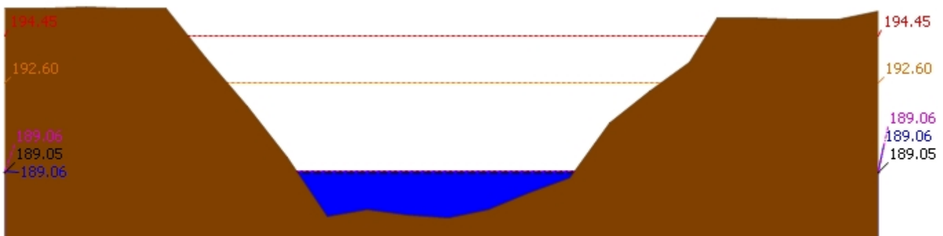
▲ ระดับปัจจุบัน --- ระดับวิกฤติ --- ระดับเฝ้าระวัง ---- เมื่อวาน 7:00 น. - - - - คาดการณ์ล่วงหน้า 1 วัน สถานี 120901T ห้วยมวกเหล็กที่ อ.มวกเหล็ก ต.มวกเหล็ก อ.มวกเหล็ก จ.สระบุรี ระดับน้ำ 189.06 ม.รทก.
