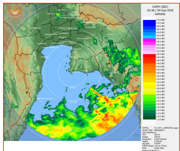
ภาพเรดาร์ตรวจอากาศ “สถานีสีตหีบ” ณ วันที่ 4 กันยายน 2561 เวลา 09.48 น. (ที่มา : กรมอุตุนิยมวิทยา)
