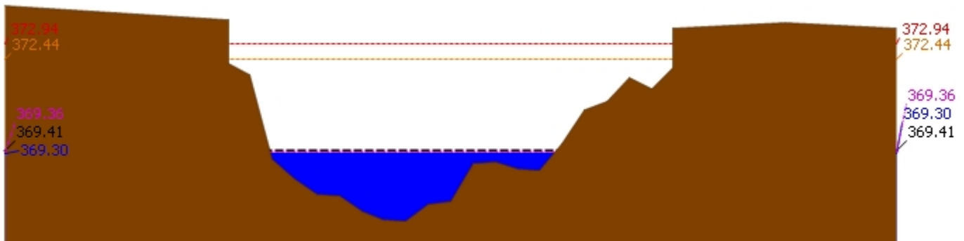
สถานี 060109T แม่น้ำปิงที่บ้านสบฮ้อ ต.แม่ระ อ.เชียงดาว จ.เชียงใหม่ ระดับน้ำ 369.30 ม.รทก.
