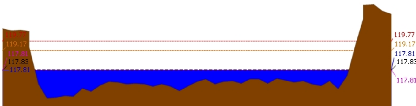
▲ ระดับปัจจุบัน --- ระดับวิกฤติ --- ระดับเฝ้าระวัง ---- เมื่อกวาน 7:00 น. - - - - คาดการณ์ล่วงหน้า 1 วัน สถานี 060111T แม่น้ำปิงที่บ้านปากร่องห้วยจี่ ต.ตากออก อ.บ้านตาก จ.ตาก ระดับน้ำ 117.81 ม.รทก.
