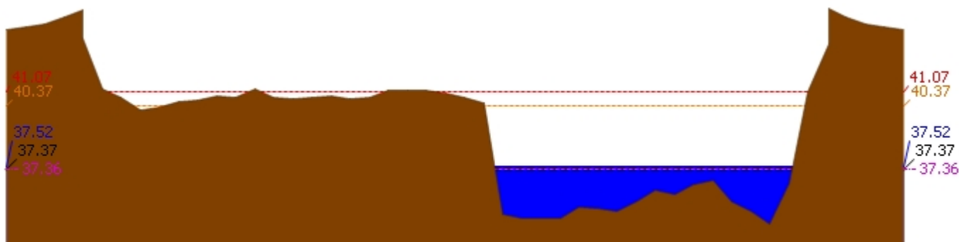
▲ ระดับปัจจุบัน --- ระดับวิกฤติ --- ระดับเฝ้าระวัง ---- เมื่อกวาน 7:00 น. - - - - คาดการณ์ล่วงหน้า 1 วัน สถานี 060110T แม่น้ำปิงที่บ้านบางแก้ว ต.บางแก้ว อ.บรรพตพิสัย จ.นครสวรรค์ ระดับน้ำ 37.52 ม.รทก.
