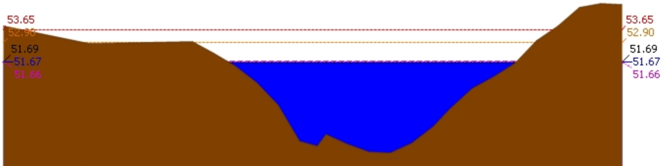
▲ ระดับปัจจุบัน --- ระดับวิกฤติ --- ระดับเฝ้าระวัง ---- เมื่อวาน 7:00 น. - - - - - คาดการณ์ล่วงหน้า 1 วัน สถานี 120113T แม่น้ำป่าสักที่บ้านเขาค้าง ต.คลองกระจิง อ.ศรีเทพ จ.เพชรบูรณ์ ระดับน้ำ 51.67 ม.รทก.
