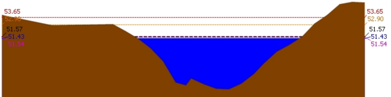
▲ ระดับปัจจุบัน --- ระดับวิกฤติ --- ระดับเฝ้าระวัง ---- เมื่อวาน 7:00 น. - - - - - คาดการณ์ล่วงหน้า 1 วัน สถานี 120113T แม่น้ำป่าสักที่บ้านเขาค้าง ต.คลองกระจิง อ.ศรีเทพ จ.เพชรบูรณ์ ระดับน้ำ 51.43 ม.รทก.
