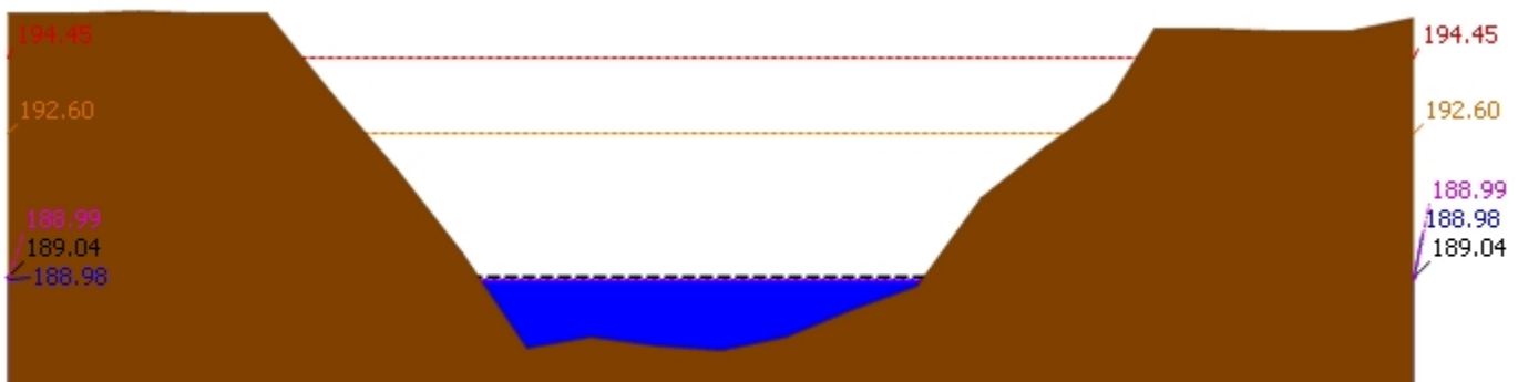
▲ ระดับปัจจุบัน --- ระดับวิกฤติ --- ระดับเฝ้าระวัง ---- เมื่อวาน 7:00 น. - - - - - คาดการณ์ล่วงหน้า 1 วัน สถานี 120901T ห้วยมวกเหล็กที่ อ.มวกเหล็ก ต.มวกเหล็ก อ.มวกเหล็ก จ.สระบุรี ระดับน้ำ 188.98 ม.รทก.
