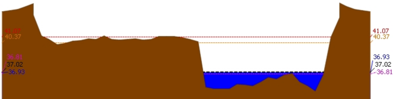
▲ ระดับปัจจุบัน --- ระดับวิกฤติ --- ระดับเฝ้าระวัง ---- เมื่อวาน 7:00 น. - - - - - คาดการณ์ล่วงหน้า 1 วัน สถานี 060110T แม่น้ำปิงที่บ้านบางแก้ว ต.บางแก้ว อ.บรรพตพิสัย จ.นครสวรรค์ ระดับน้ำ 36.93 ม.รทก.
