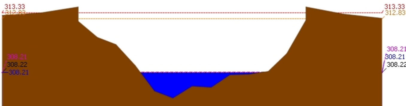
▲ ระดับปัจจุบัน --- ระดับวิกฤติ --- ระดับเฝ้าระวัง ---- เมื่อวาน 7:00 น. - - - - - คาดการณ์ล่วงหน้า 1 วัน สถานี 060814T น้ำแม่ฆานที่บ้านท่าโป่ง ต.บ้านแม อ.สันป่าตอง จ.เชียงใหม่ ระดับน้ำ 308.21 ม.รทก.
