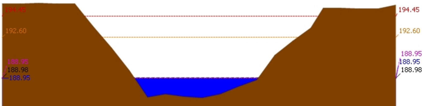
▲ ระดับปัจจุบัน --- ระดับวิกฤติ --- ระดับเฝ้าระวัง ---- เมื่อกวาน 7:00 น. - - - - คาดการณ์ล่วงหน้า 1 วัน สถานี 120901T ห้วยมวกเหล็กที่ อ.มวกเหล็ก ต.มวกเหล็ก อ.มวกเหล็ก จ.สระบุรี ระดับน้ำ 188.95 ม.รทก.
