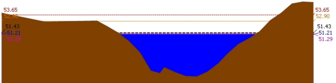
▲ ระดับปัจจุบัน --- ระดับวิกฤติ --- ระดับเฝ้าระวัง ---- เมื่อกวาน 7:00 น. - - - - คาดการณ์ล่วงหน้า 1 วัน สถานี 120113T แม่น้ำป่าสักที่บ้านเขาค้าง ต.คลองกระจิง อ.ศรีเทพ จ.เพชรบูรณ์ ระดับน้ำ 51.21 ม.รทก.
