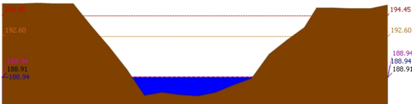
▲ ระดับปัจจุบัน --- ระดับวิกฤติ --- ระดับฝายระวัง ---- เมื่อวาน 7:00 น. - - - - - คาดการณ์ล่วงหน้า 1 วัน สถานี 120901T ห้วยมวกเหล็กที่ อ.มวกเหล็ก ต.มวกเหล็ก อ.มวกเหล็ก จ.สระบุรี ระดับน้ำ 188.94 ม.รทก.
