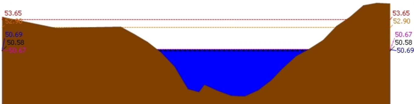
▲ ระดับปัจจุบัน --- ระดับวิกฤติ --- ระดับเฝ้าระวัง ---- เมื่อวาน 7:00 น. - - - - - คาดการณ์ล่วงหน้า 1 วัน สถานี 120113T แม่น้ำป่าสักที่บ้านเขาค้าง ต.คลองกระจิง อ.ศรีเทพ จ.เพชรบูรณ์ ระดับน้ำ 50.69 ม.รทก.
