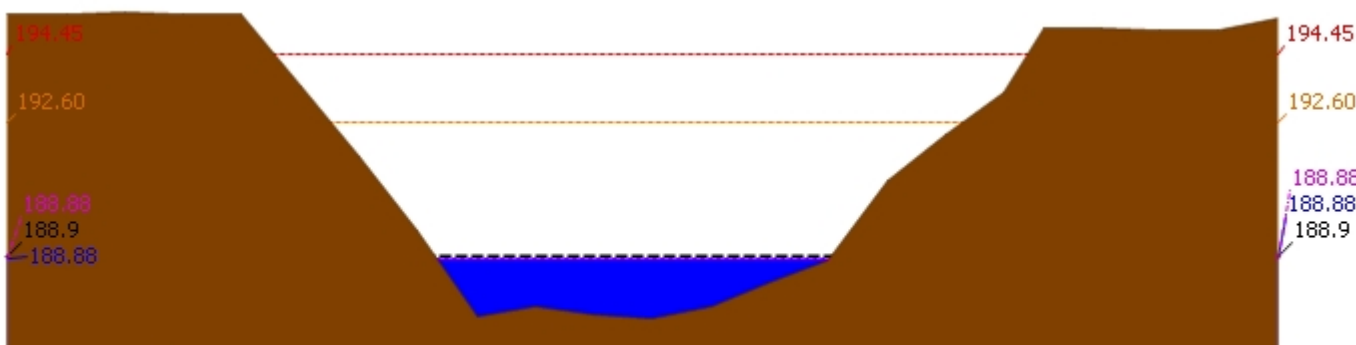
▲ ระดับปัจจุบัน --- ระดับวิกฤติ --- ระดับเฝ้าระวัง ---- เมื่อวาน 7:00 น. - - - - - คาดการณ์ล่วงหน้า 1 วัน สถานี 120901T ห้วยมวกเหล็กที่ อ.มวกเหล็ก ต.มวกเหล็ก อ.มวกเหล็ก จ.สระบุรี ระดับน้ำ 188.88 ม.รทก.
